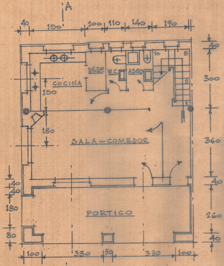
B. Planta
