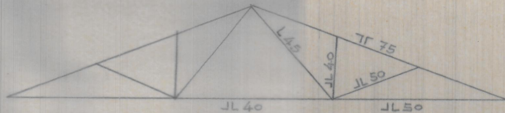
Armadura ESCALA=1:100
