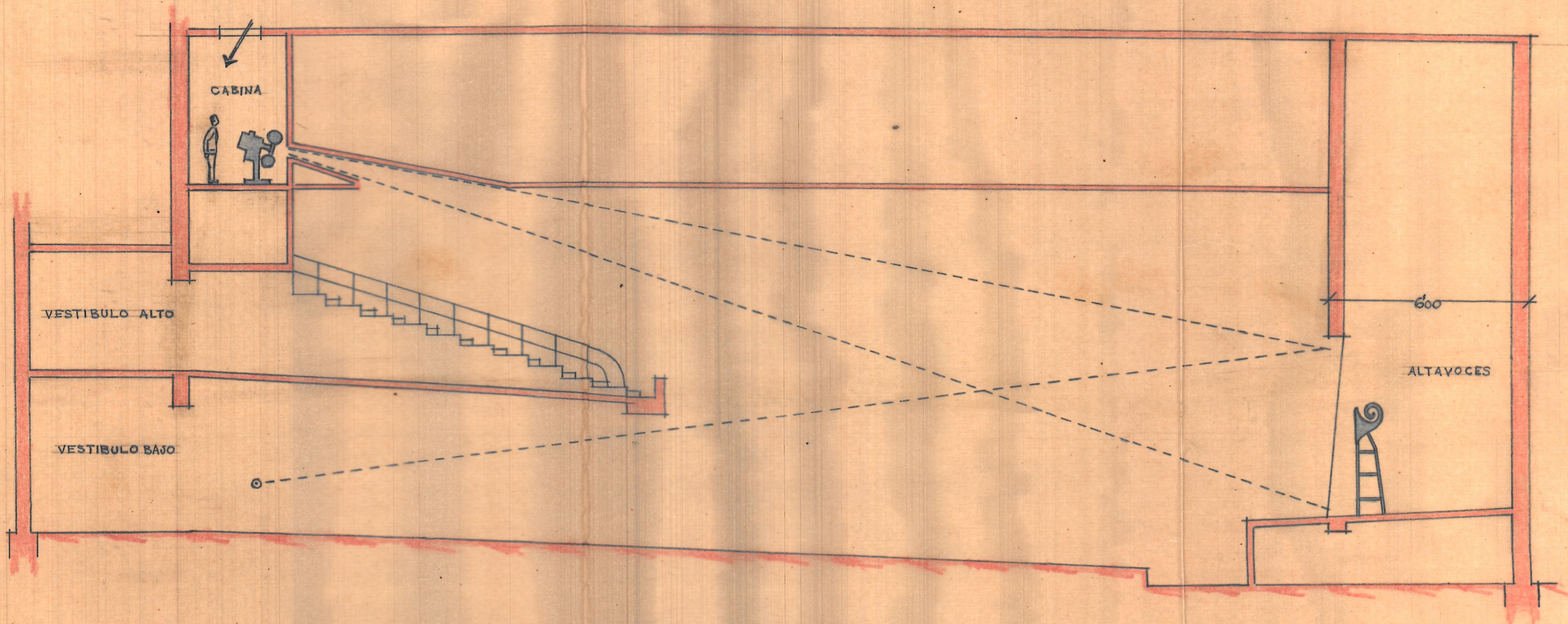
Sección longitudinal de la reforma proyecto ESCALA = 1:100
