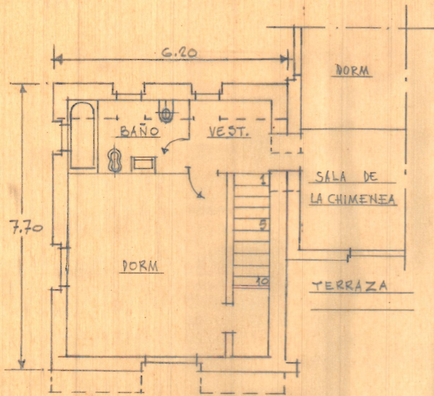
Planta baja
