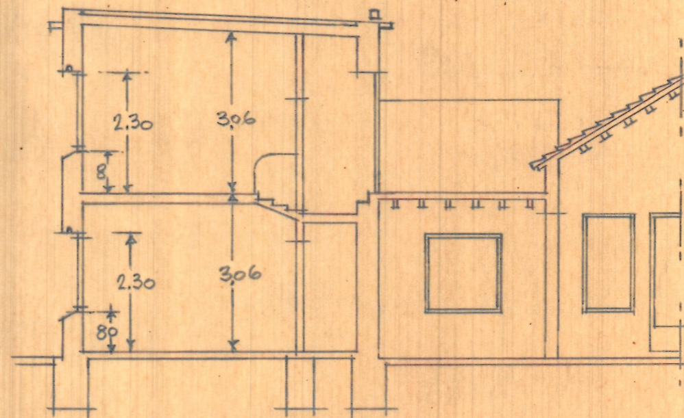
Sección transversal
