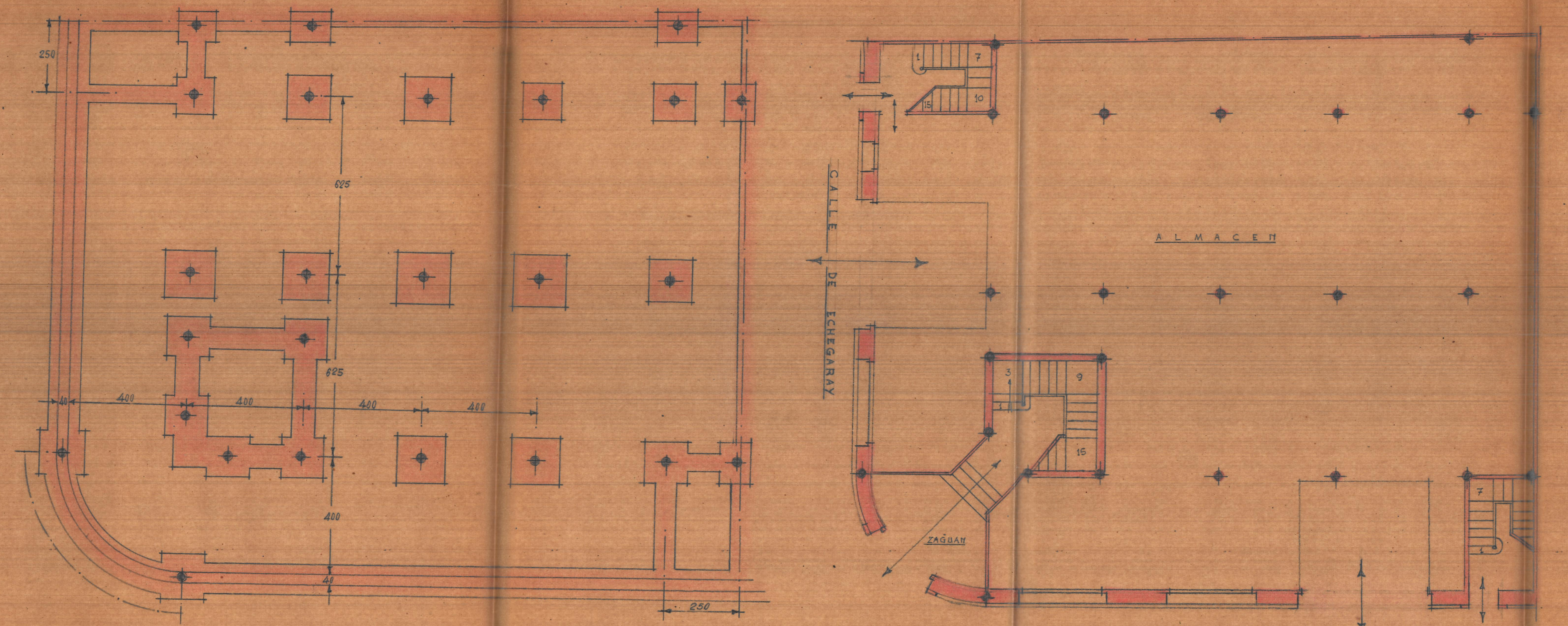
Planta de cimentación
