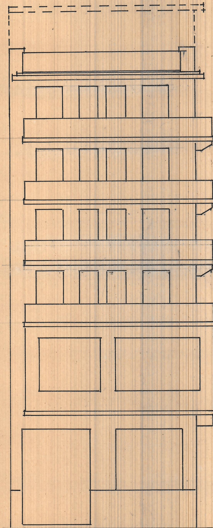
FACHADA A LA CALLE DEL JAY-ALAY — E-1:100
