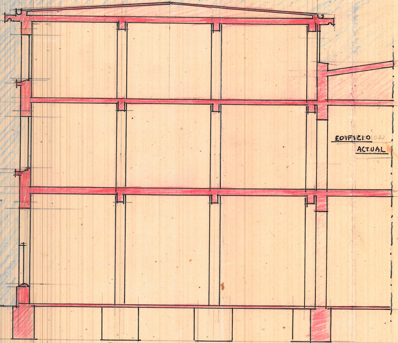
SECCION A-B
