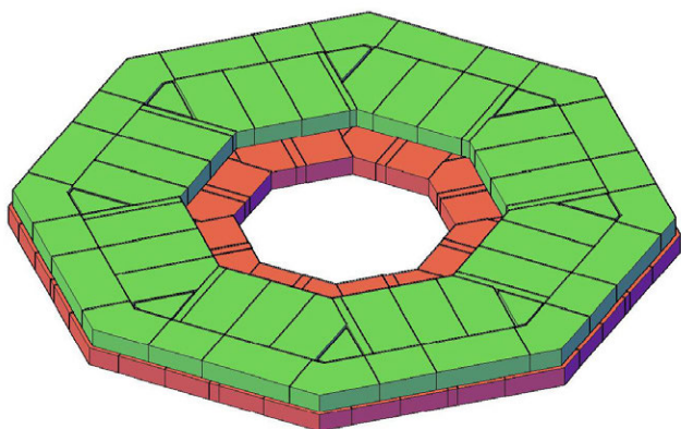
Figura 9. Montaje de una sección octogonal con piezas aplanilladas y escalón interior.
