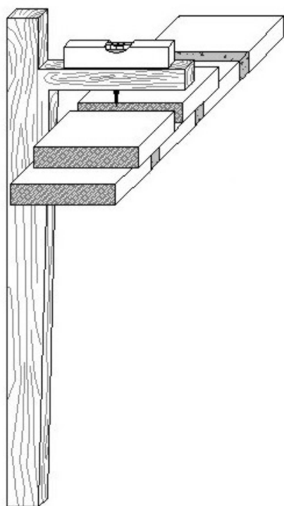
Figura 10. Taulaplom.
