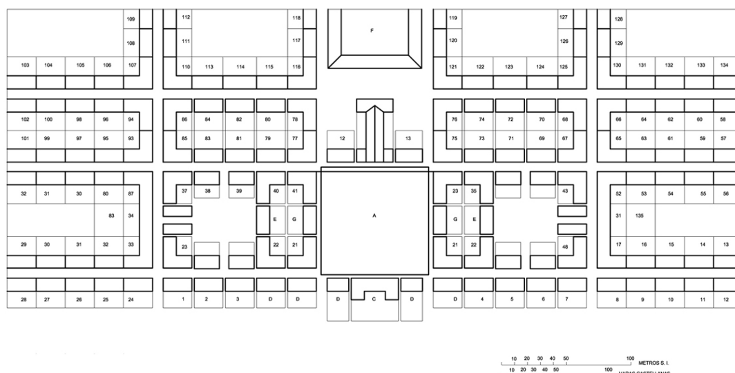
FIGURA 4. PROYECTO DE BERANGER PARA LA NUEVA POBLACIÓN DE SAN CARLOS (1768) (PROYECTO DE NUEVA POBLACIÓN EN LA PUNTA DE TECQUE, DE LA ISLA DE CHILOÉ. CHACAO, 6 DE SEPTIEMBRE DE 1768. BC, MS. 400, N°1). SE TRANSFORMA EL MODELO CLÁSICO DE POBLACIÓN INDIANO. AUNQUE SE MANTIENE LA PLAZA CUADRANGULAR Y EL TRAZADO RECTILÍNEO DE LAS CALLES, LAS MANZANAS SON RECTANGULARES Y DE PROPORCIONES DIVERSAS. LOS LOTES DE PROPIEDAD SON MENORES Y MENOS GENEROSOS QUE LOS CUARTOS DE MANZANA DEL URBANISMO PRECEDENTE.
