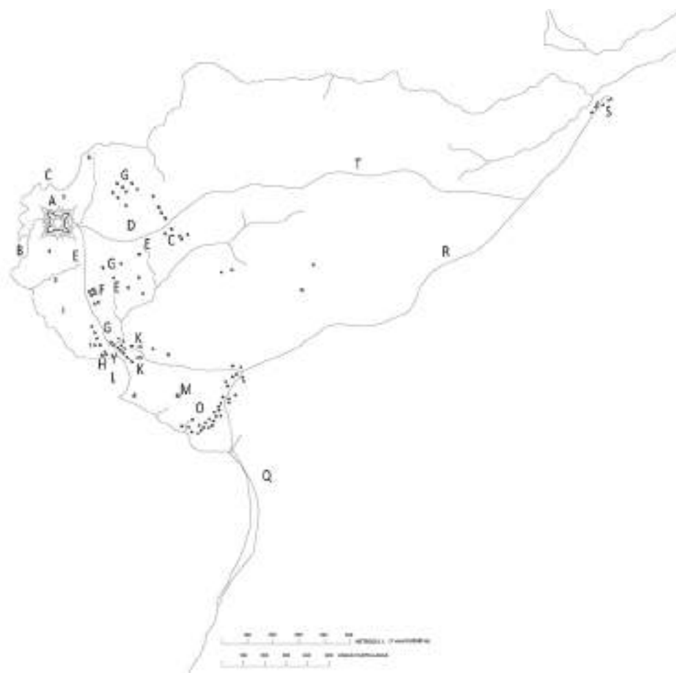
FIGURA 2. PLANO DE SITUACIÓN DEL FUERTE REAL DE SAN CARLOS Y CONSTRUCCIONES ALEDAÑAS FIRMADO POR CARLOS DE BERANGER EL 28 DE DICIEMBRE DE 1769 (CGE, AR. J-T.9-C.1-133).
