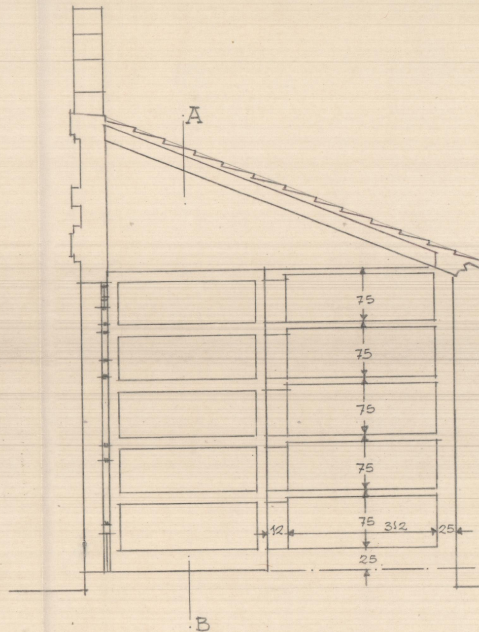
Sección longitudinal
