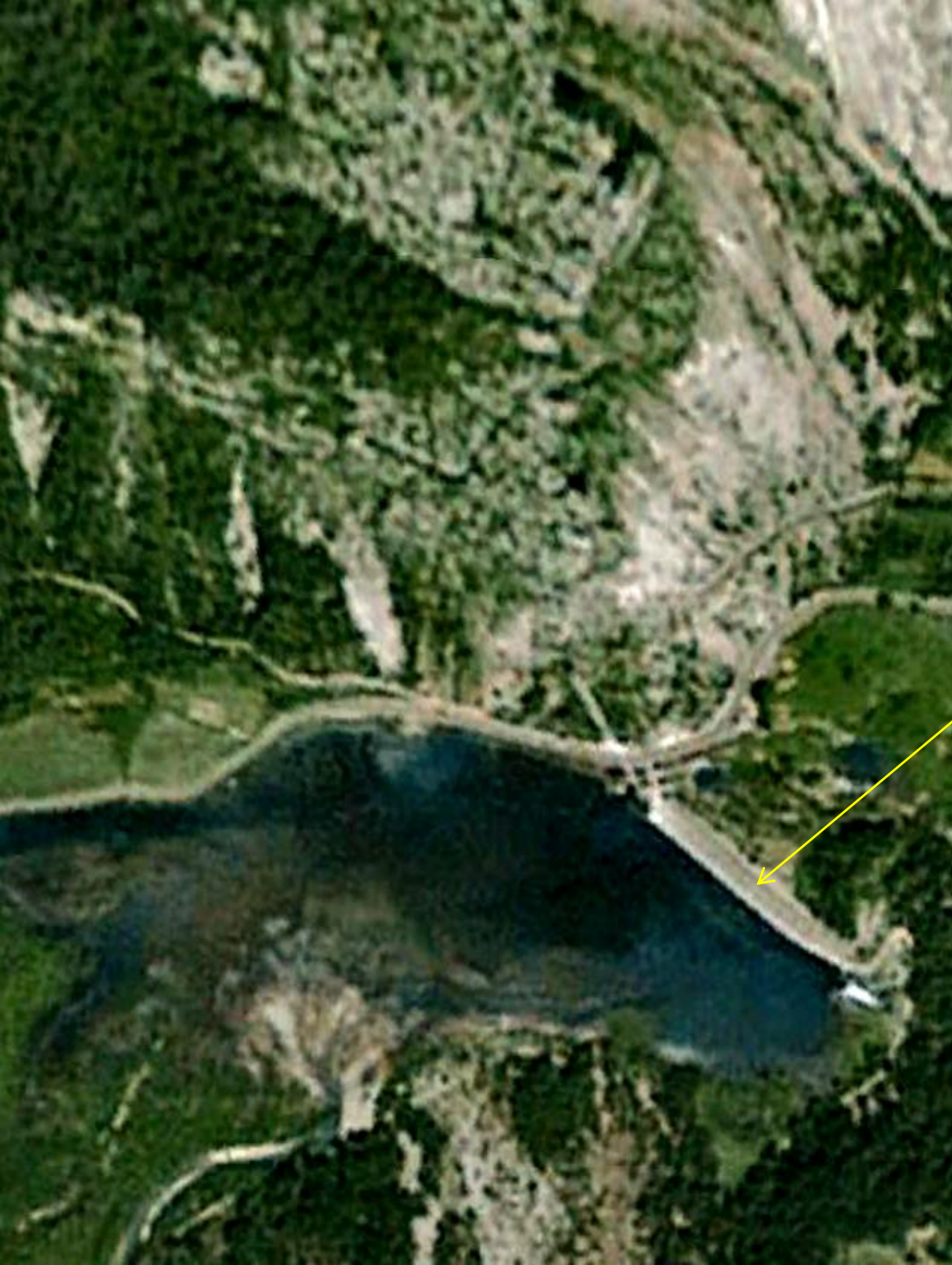
Embalse de Pineta. W de Bielsa. NW Hoja. (por Gonzalo Martinez Hernandez- Google)
