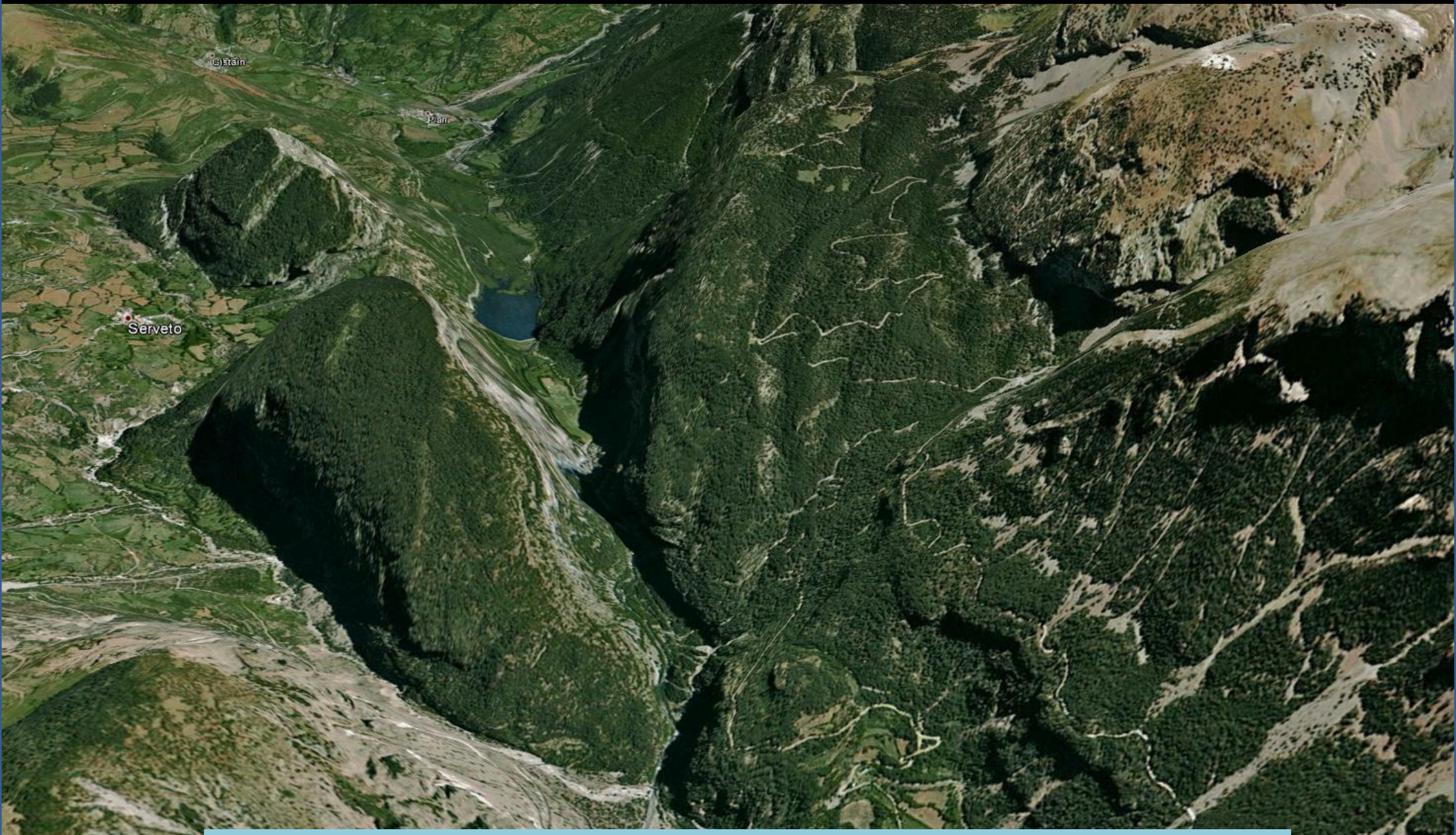
Perspectiva desde el W, relieve realizado, del Valle del Río Cinqueta, el Embalse de Plandescún. A izq., del valle, Peñas de Arties, Serveto, y De Sin, Terciarios. Centro Hoja de Bielsa. A der. Paso de La Inclusa, Terciario, cabalgamientos, y Collado de Ibón, Cretácico Sup.
