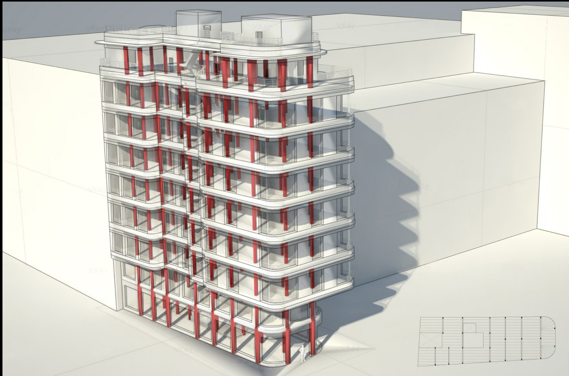
Esquema estructura
