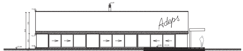
Alzado este / Restaurante East Elevation / Restaurant
