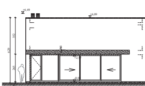
Alzado sur / Conciergerie South Elevation / Conciergerie
