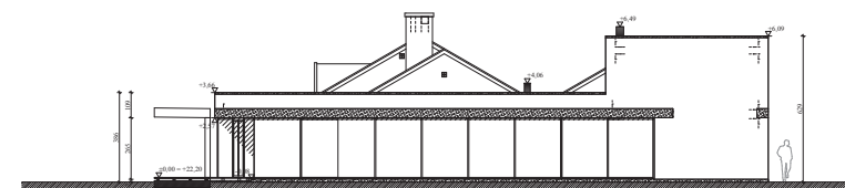
Alzado oeste / Administración y conserjería West Elevation / Administration and Caretaker's Office
