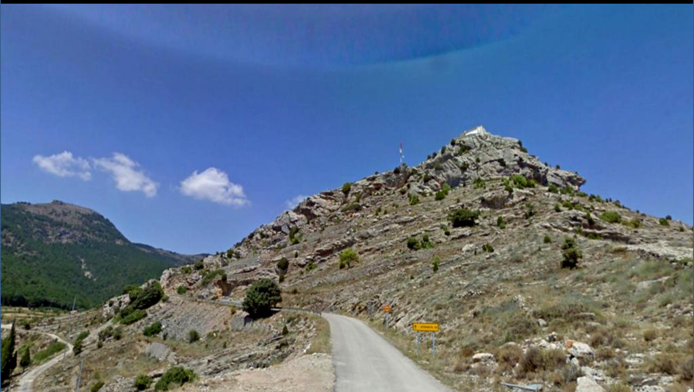
Calizas Bedouliense. Aptiense, Cretácico Inf. NW Chodos. Centro E. Hoja de Villahermosa del Río
