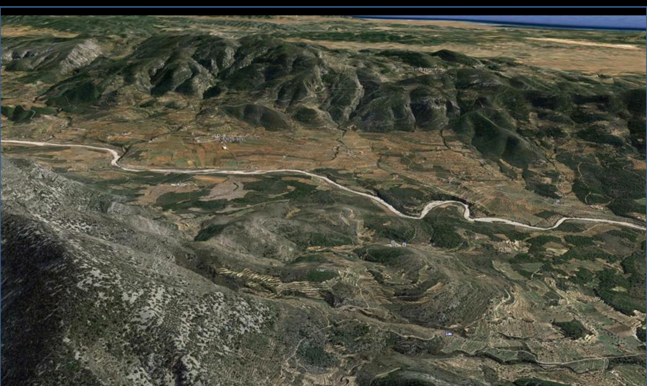
Perspectiva desde el W- relieve realzado- de la fosa de la Rambla de La Viuda. Al NW de Sierra de Engarcerán, Castellón. Entre relieves de Cretácicos. NW Hoja de Cuevas de Vinromá.
