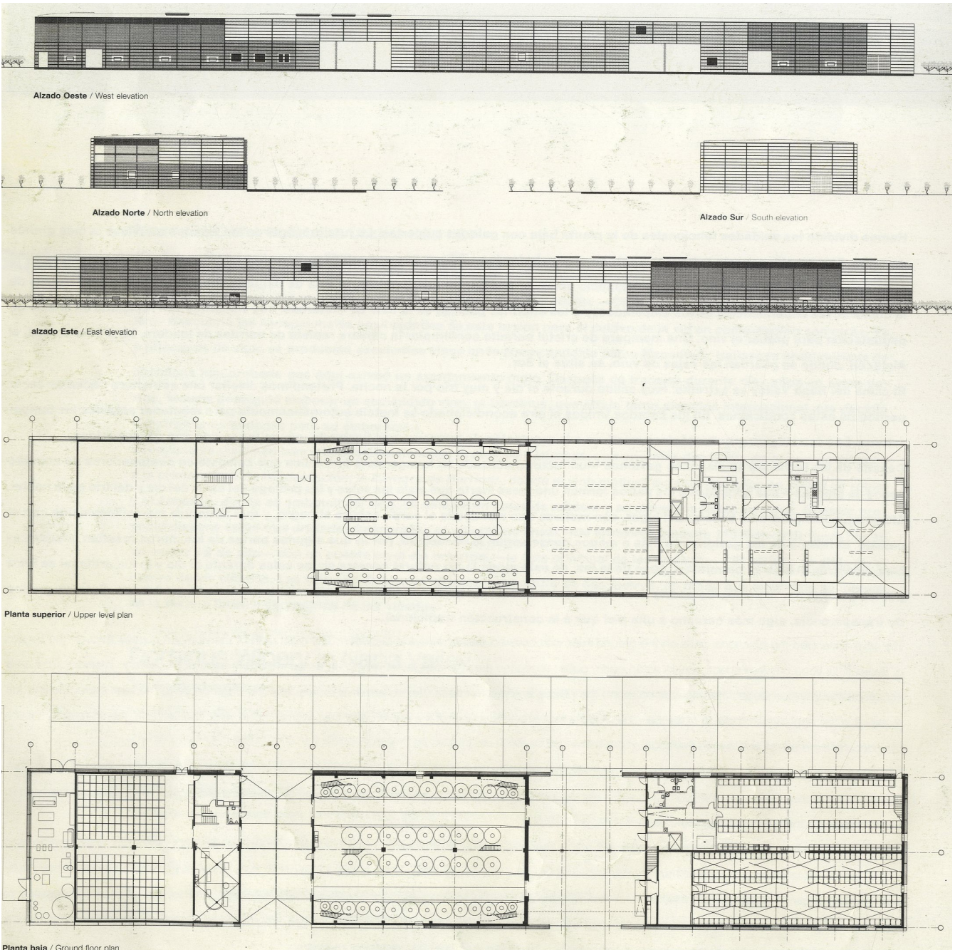
Img. 21 Plantas, Alzados y Secciones Bodegas Dominus
