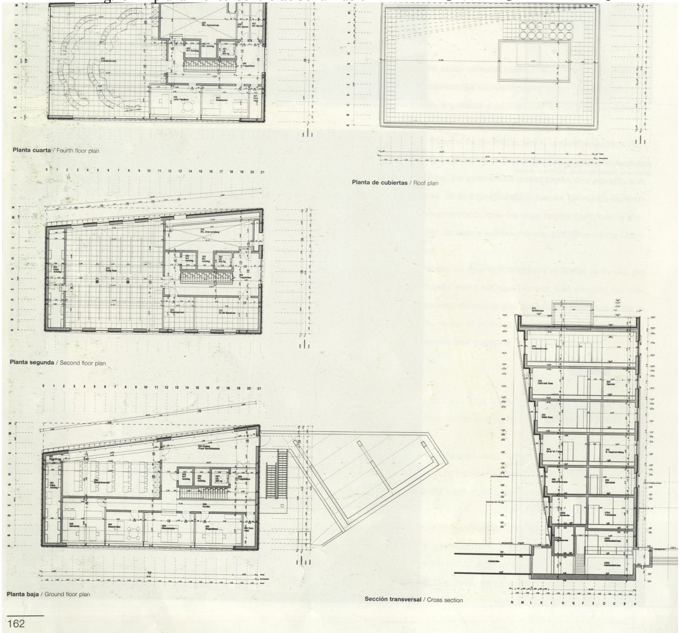
Img. 30 Plantas, y Secciones Centro de Señalización
