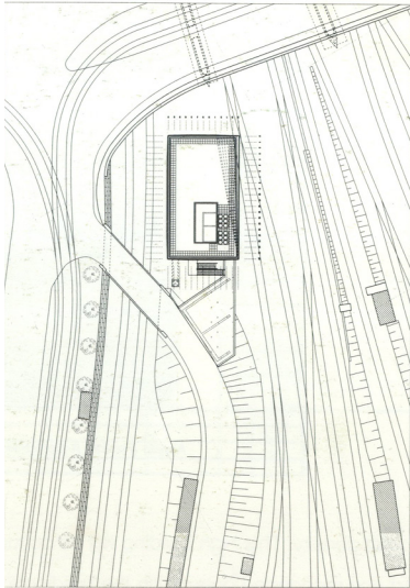
Img.28 Emplazamiento Centro de Señalización
