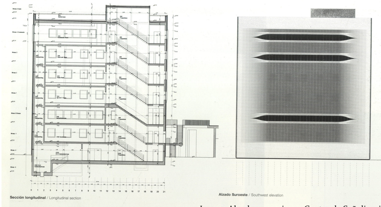
Img. 31 Alzados y secciones Centro de Señalización
