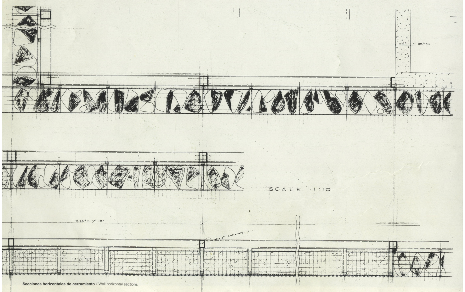
Img. 25 Plantas de detalle
