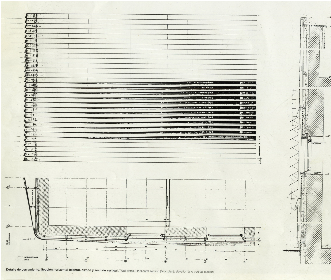
Img. 34 Planta, Alzado y Sección del Centro de Señalización
