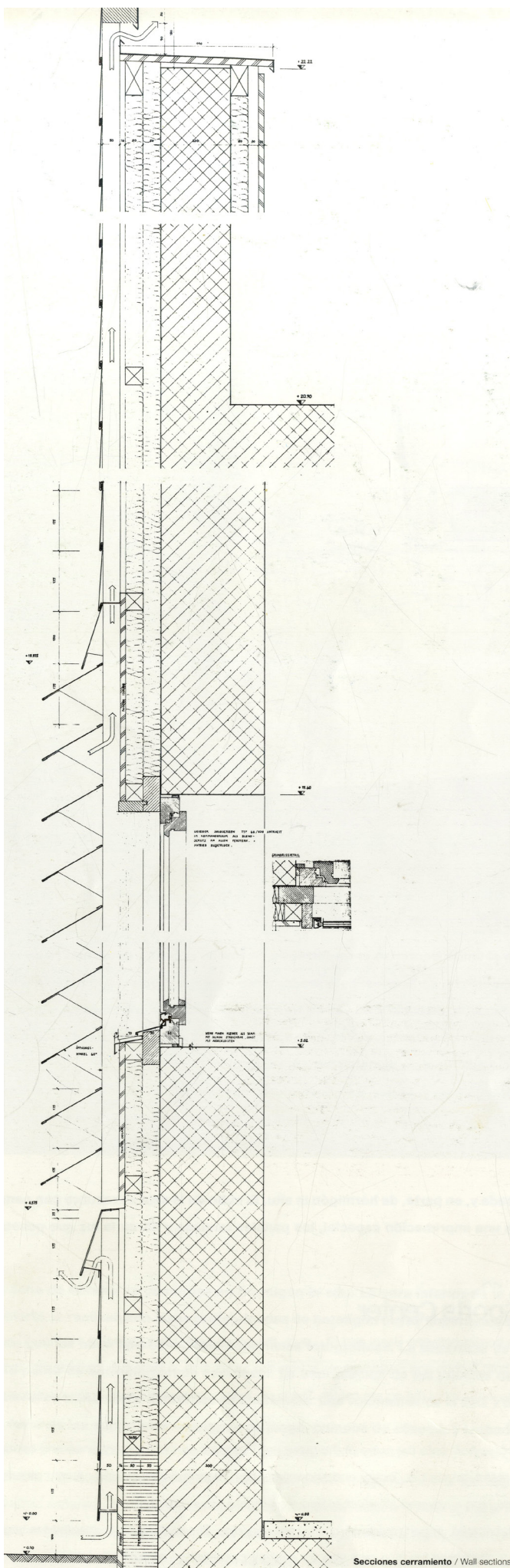
Img. 36 Sección constructiva Detalle de ventana
