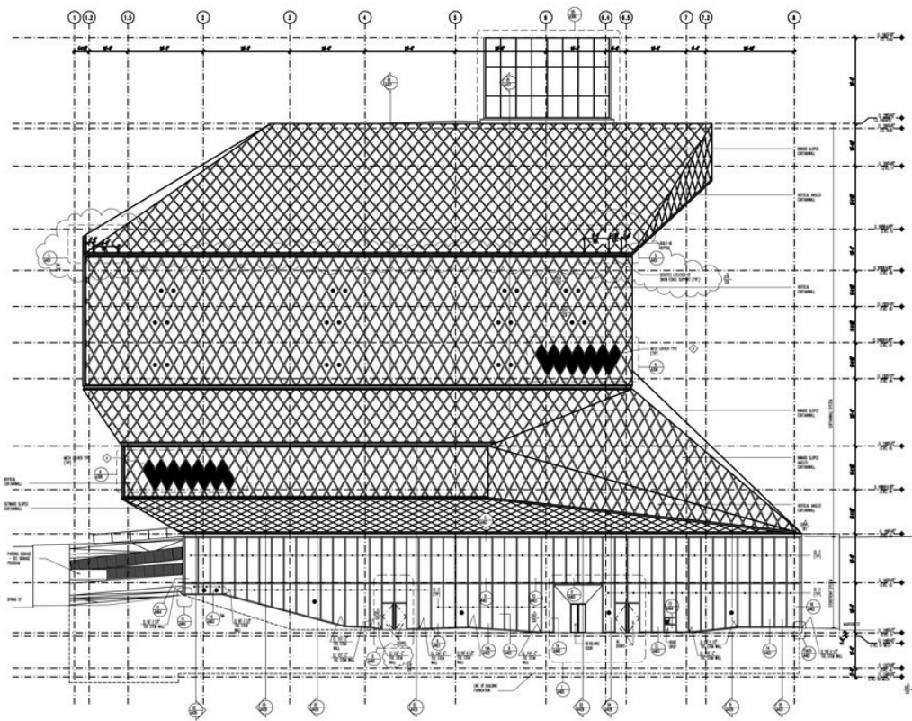
Alzado oeste
