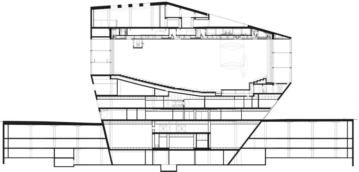
Sección longitudinal
