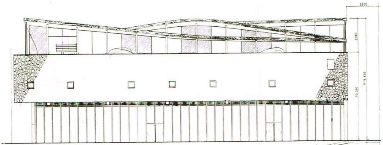
Alzado sur
