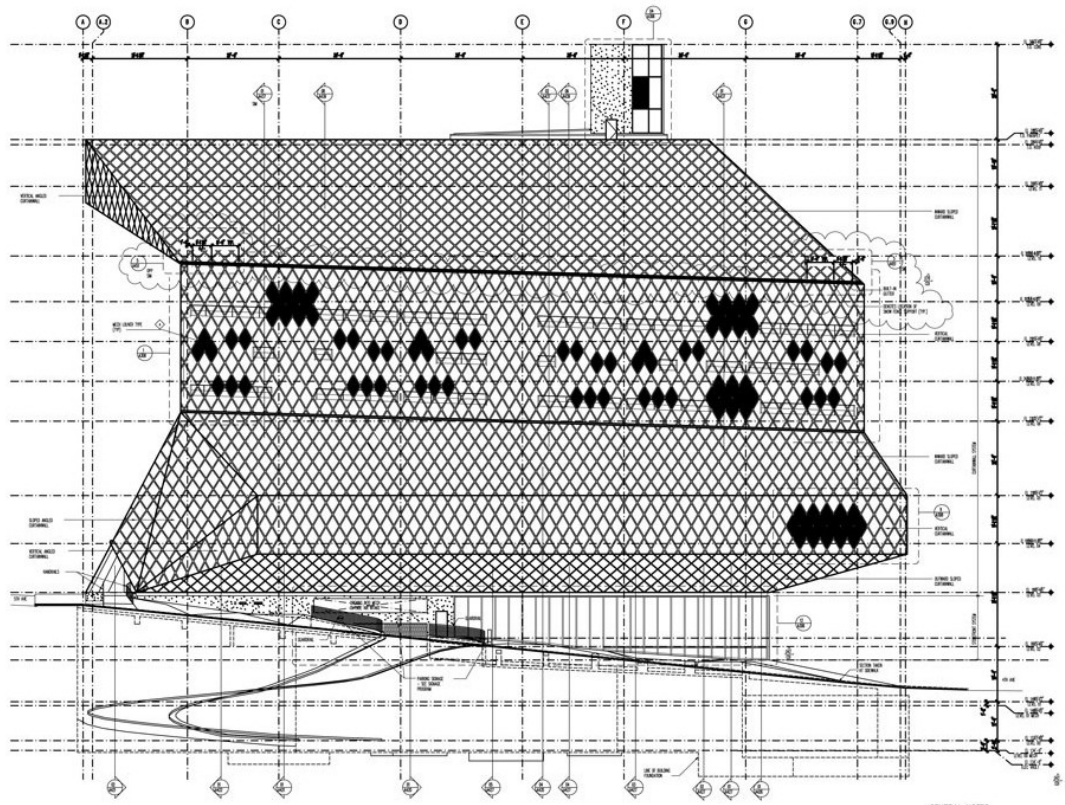
Alzado norte
