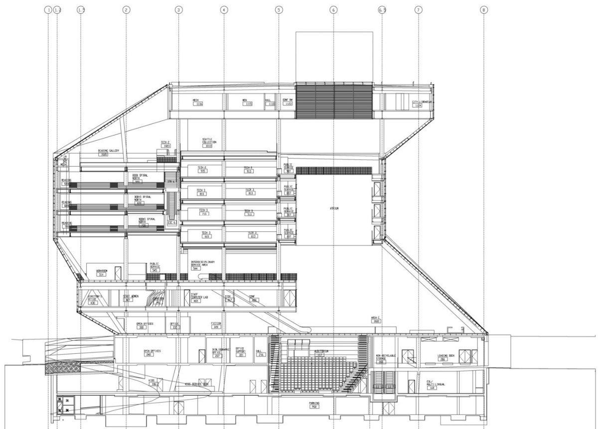
Sección transversal
