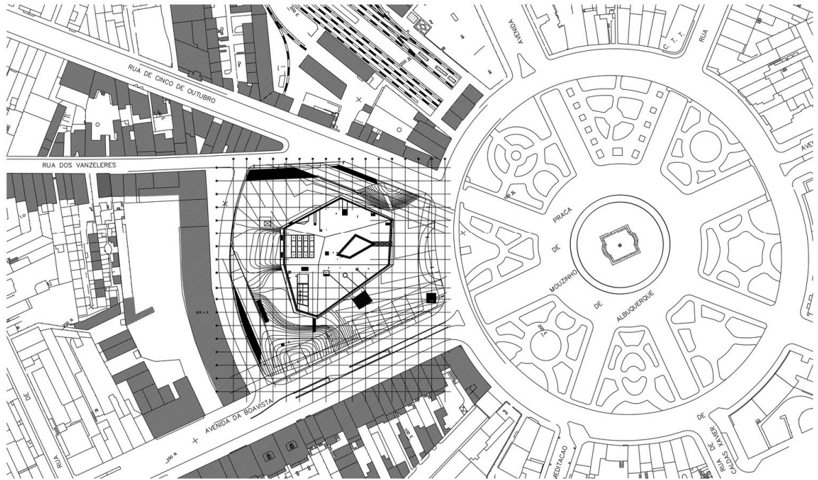
Plano localización
