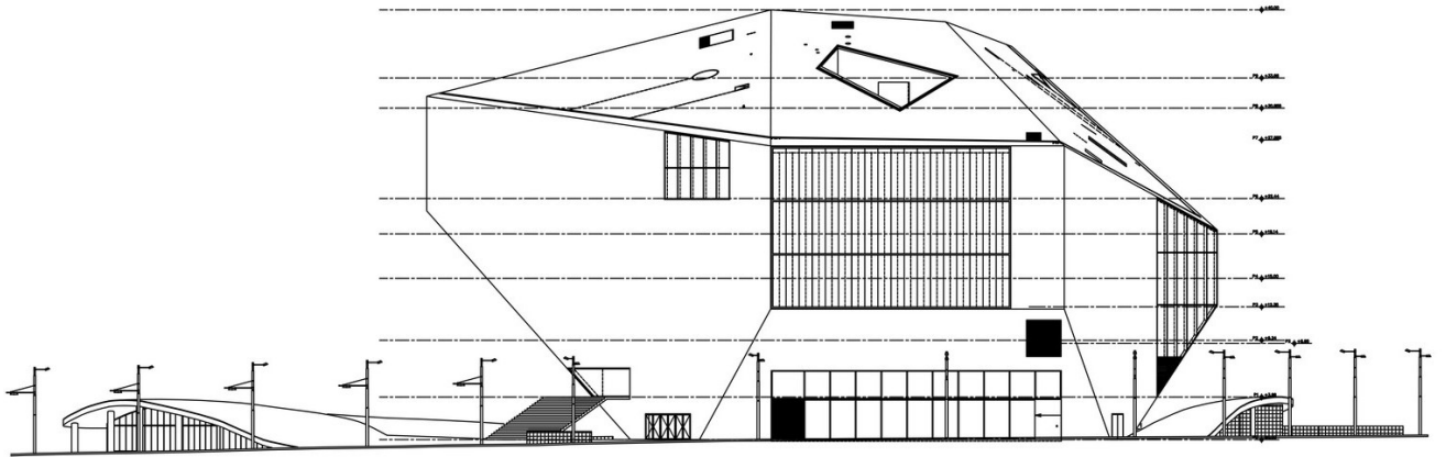
Alzado Sureste
