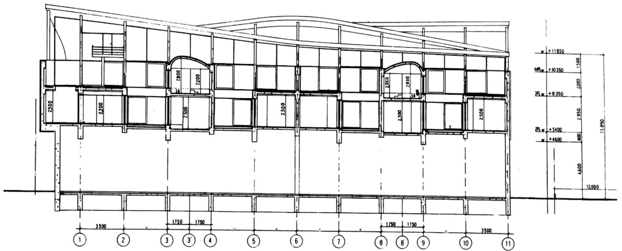
Sección longitudinal
