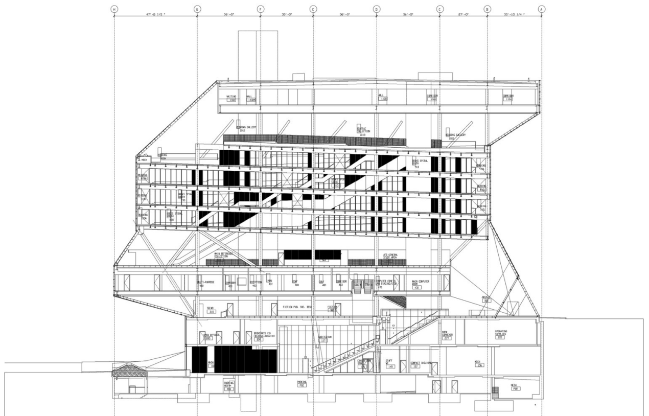
Sección longitudinal
