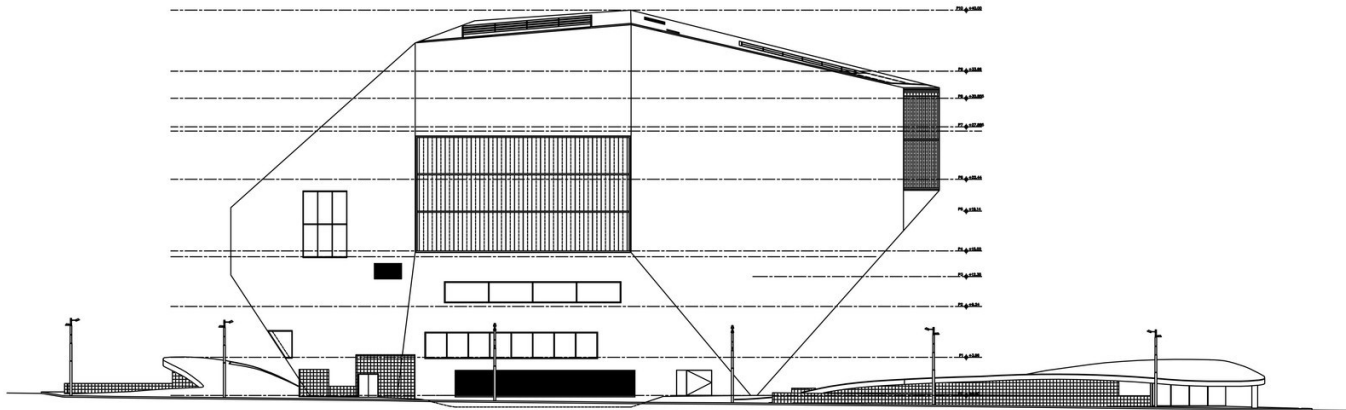
Alzado Noroeste
