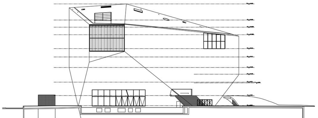
Alzado Suroeste
