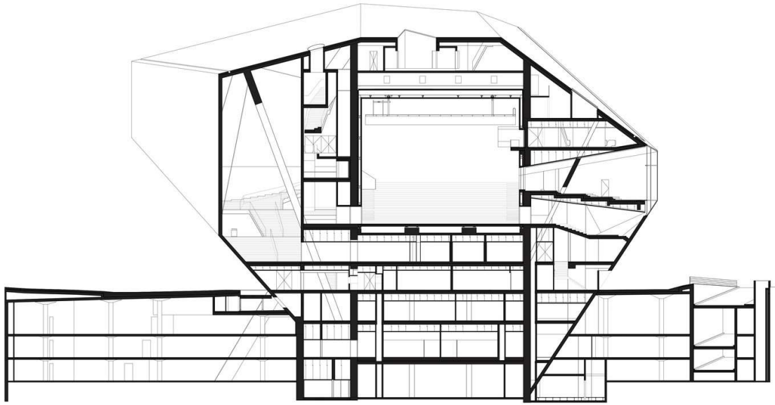
Sección transversal
