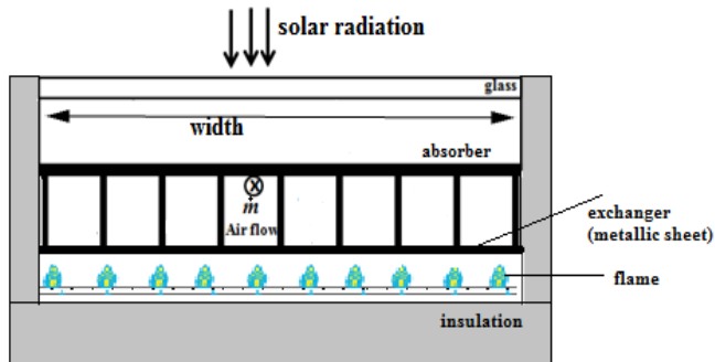
Fig. 1 Solar-gas collector.
