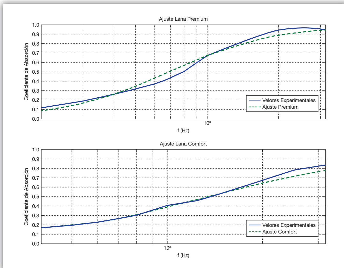
Figura 4. Resultados del ajuste propio para las lanas Premium y Comfort. (Línea continua; valores experimentales/ línea discontinua; resultados del ajuste).
