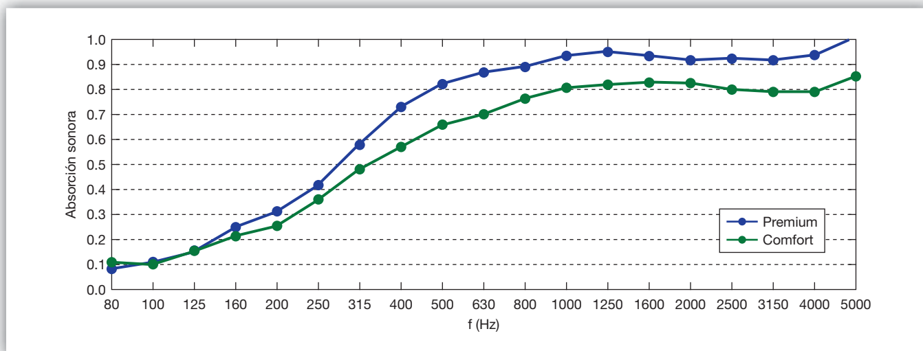
Figura 3. Absorción sonora en cámara reverberante de la EPSG-UPV según UNE EN ISO 354:2004 para las muestras Premium y Comfort.
