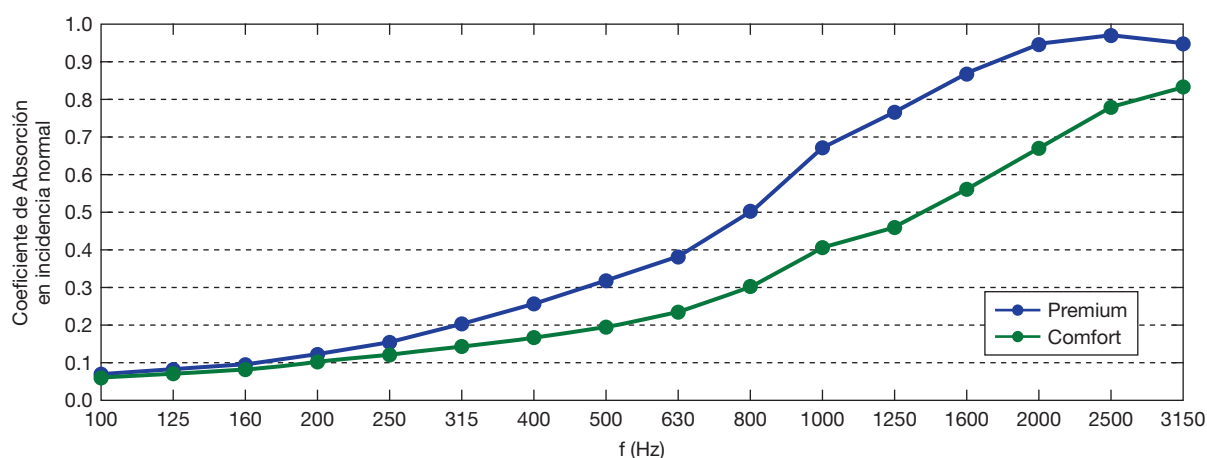
Figura 2. Coeficiente de absorción en función de la frecuencia en incidencia normal según UNE EN ISO 10534-2:2002 para las muestras Premium y Comfort.
