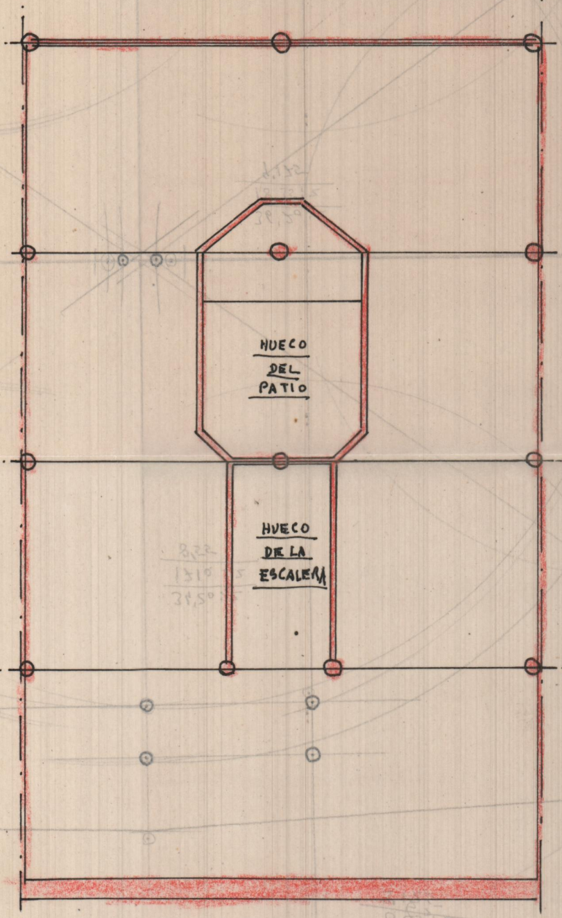
ESTRUCTURA DE PISOS Y CUBIERTA
