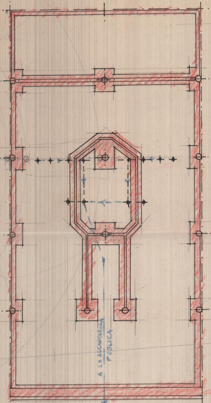
PLANTA DE CIMIENTOS Y DESAGUES
