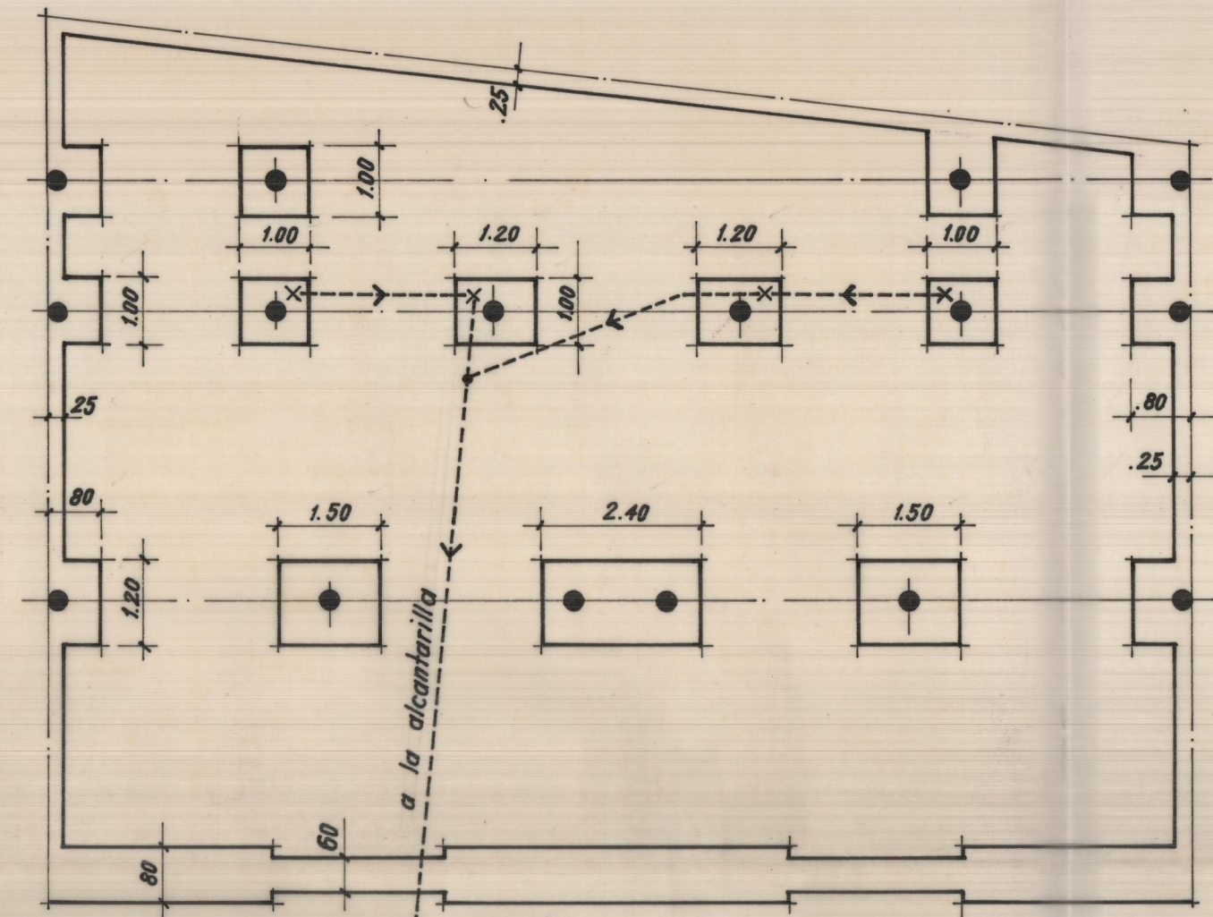
cimientos y desagües
