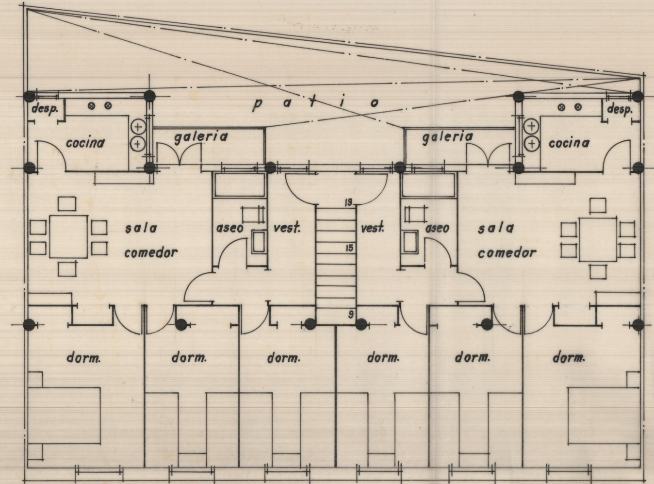
planta alta.- disposición
