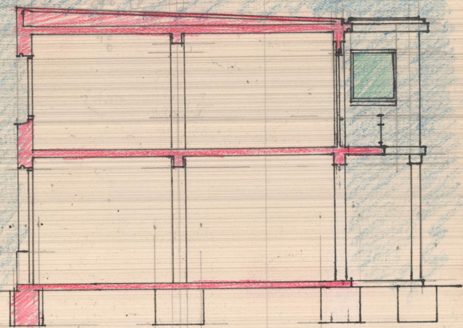
SECCION A-B
