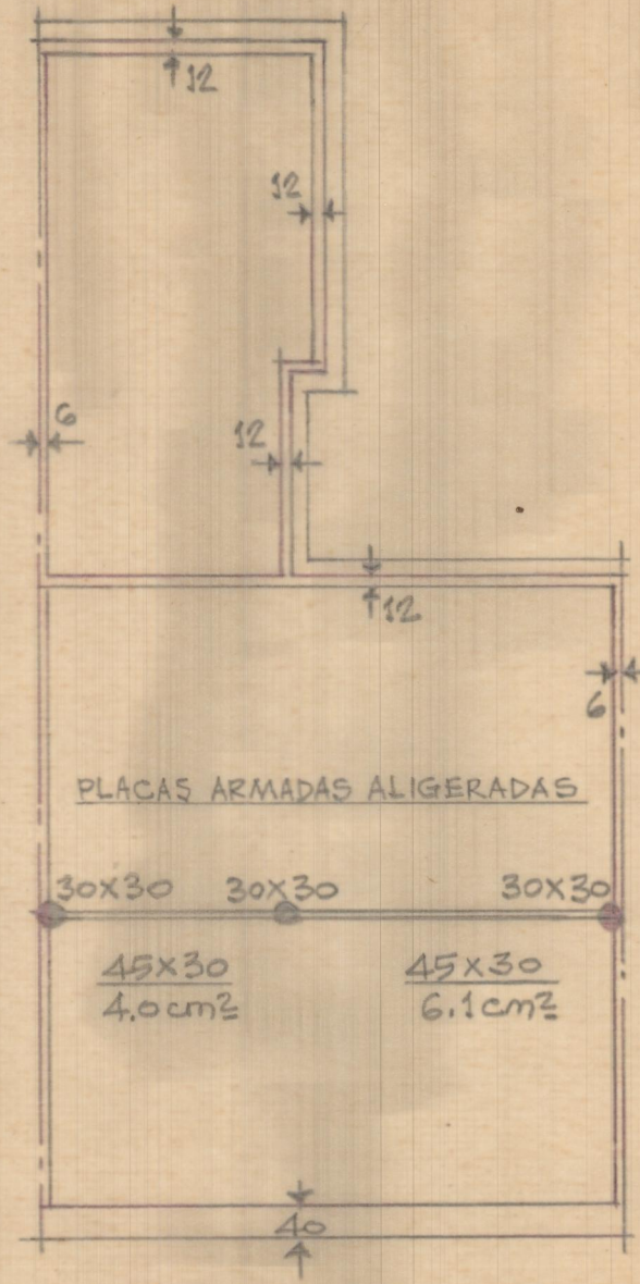
Planta de armadura y de vigas Estructura de cubierta
