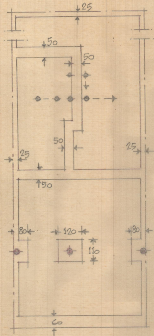
Planta de armadura y de vigas Estructura de cubierta
