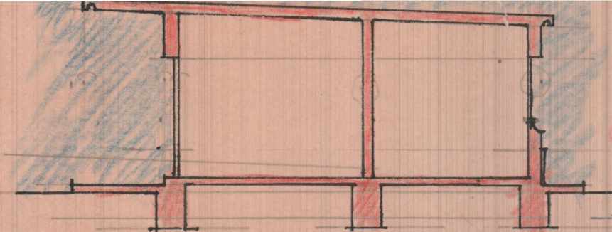
SECCION POR EL EJE 9.20
