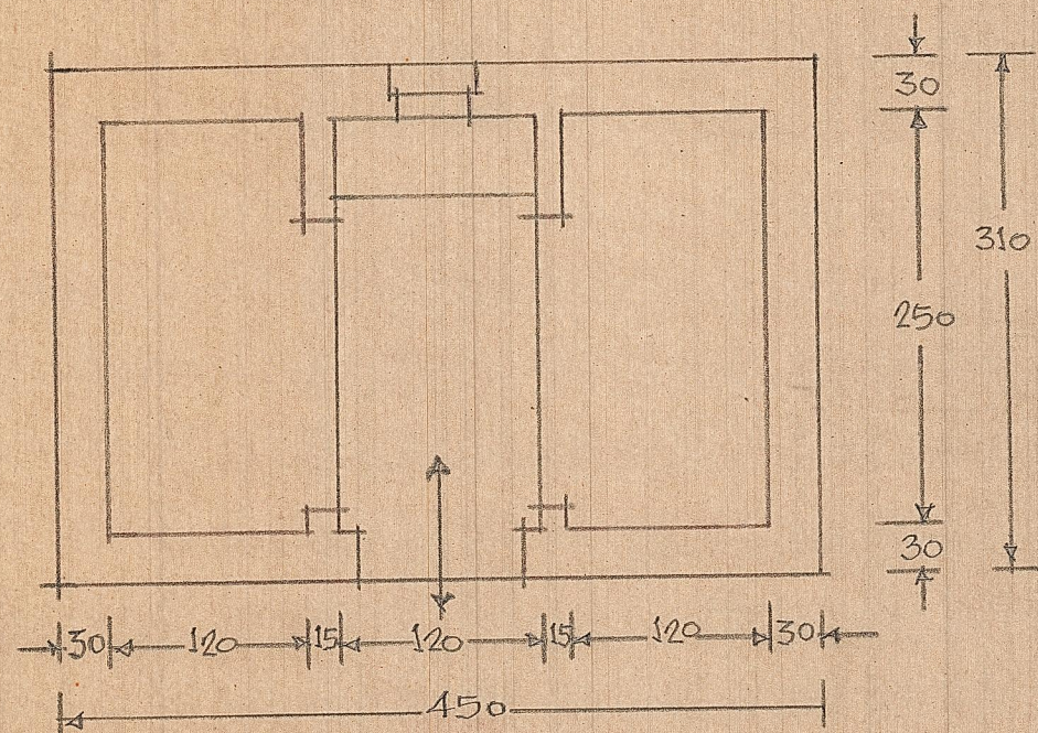
Sección horizontal por A-B.
