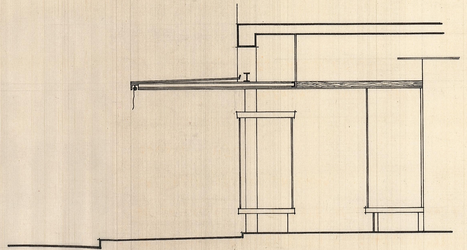
sección a.-a.
