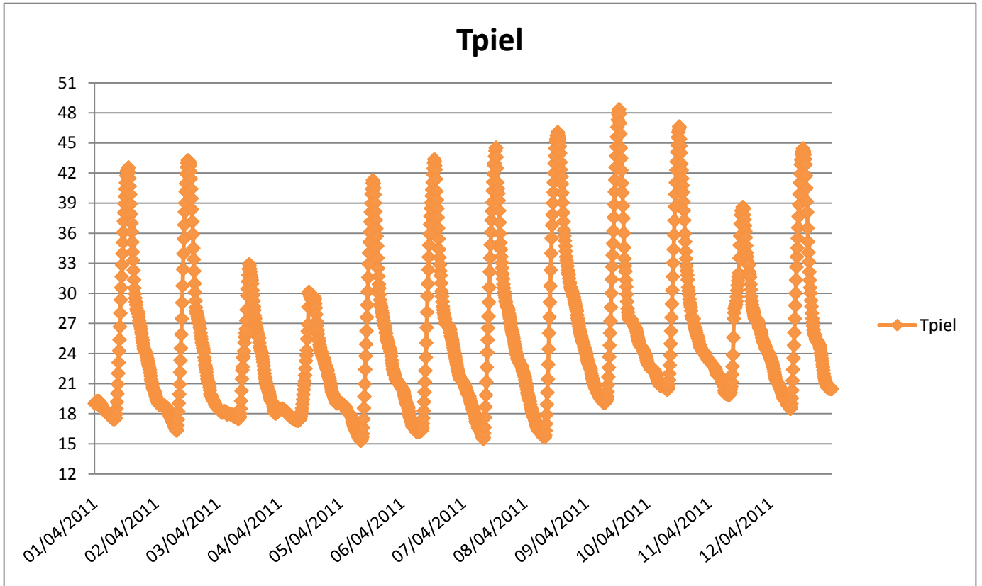
Figura 27. Gráfica de la temperatura de la capa de la piel exterior del muro.
