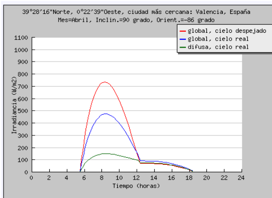
Figura 19. Radiación solar incidente sobre paramento vertical para distintas orientaciones en el mes de Abril en W/m^2 . [5]
