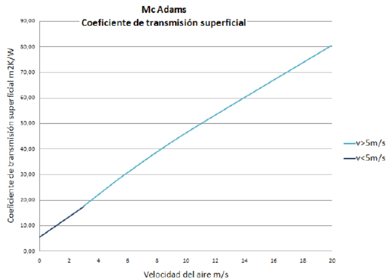
Figura 21. Gráfica con los valores de convección mixta sobre una superficie propuestos por Mc Adams. [2]
