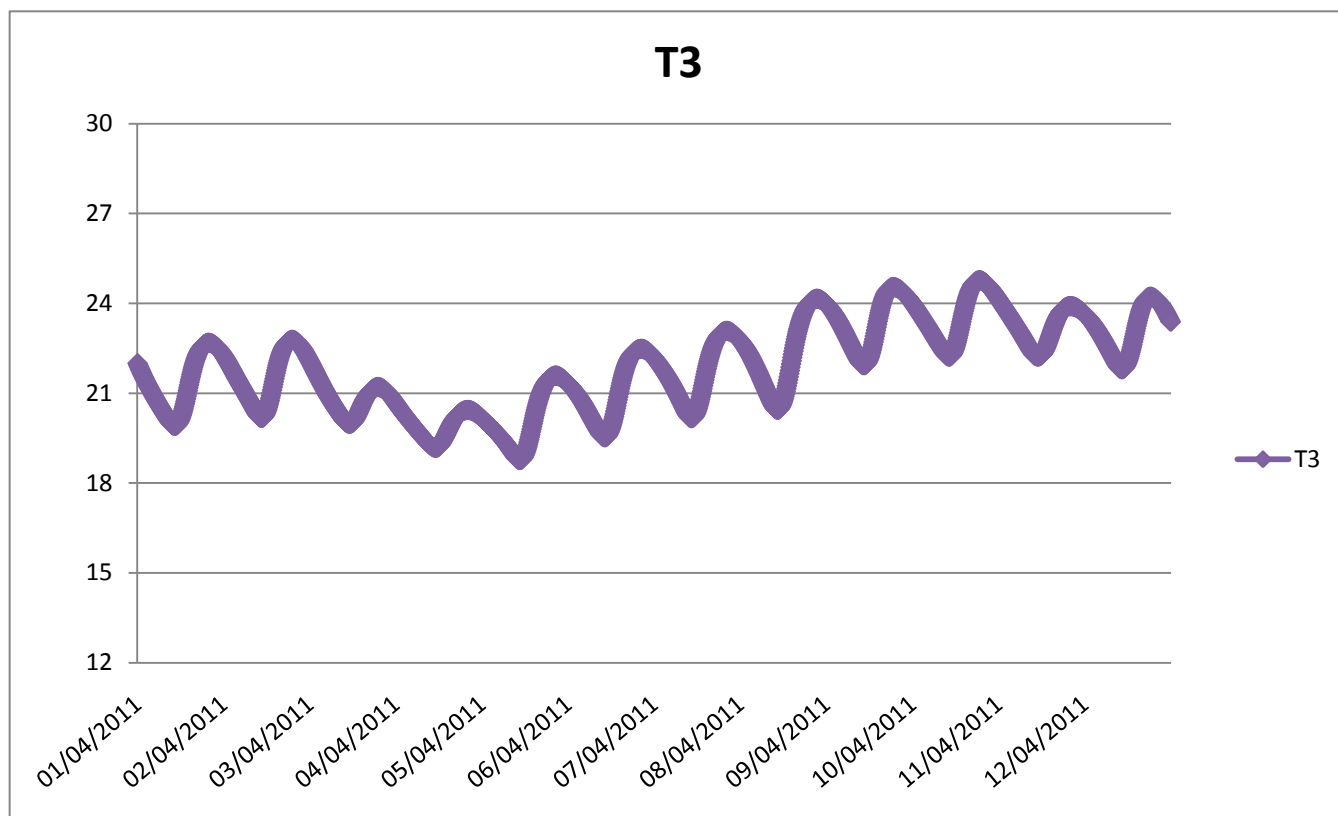
Figura 25. Gráfica de la Temperatura de la capa 3.
