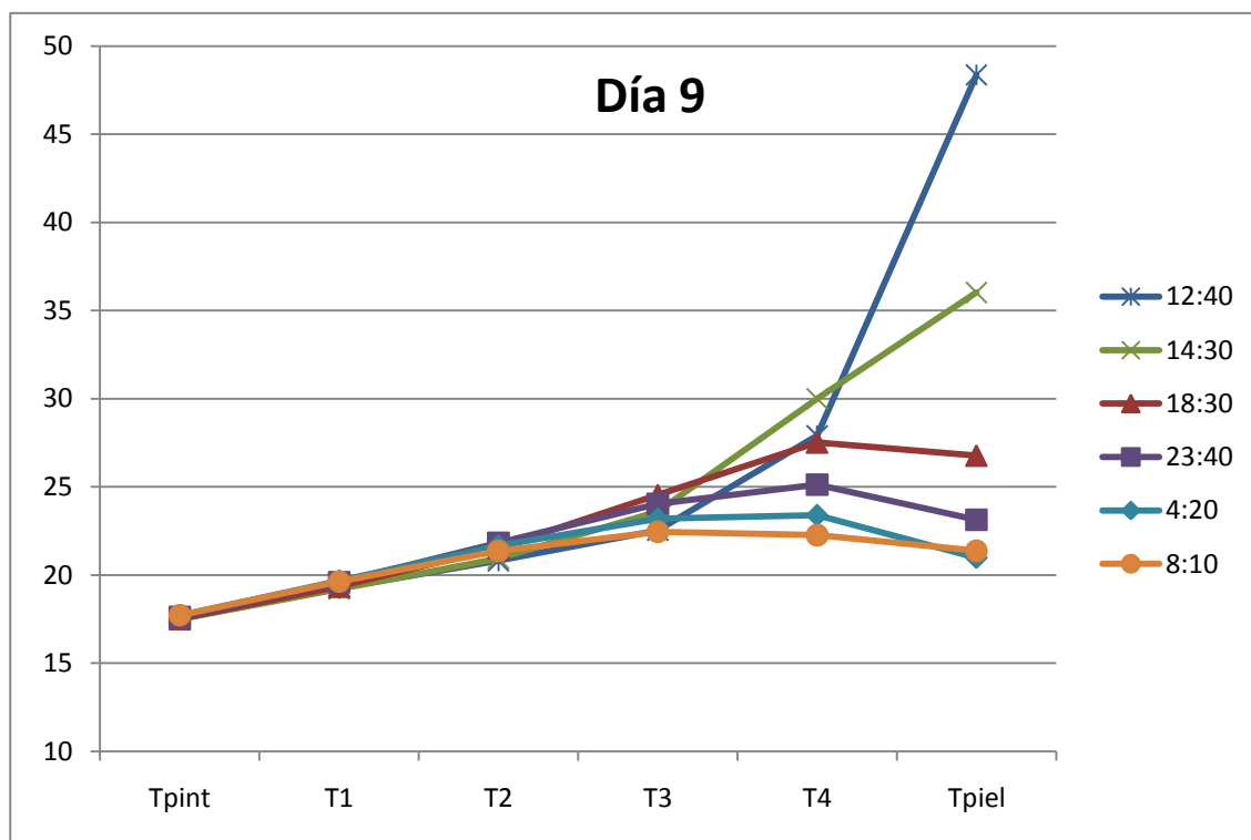
Figura 31. Gráfica del perfil térmico del cerramiento del día 9.
