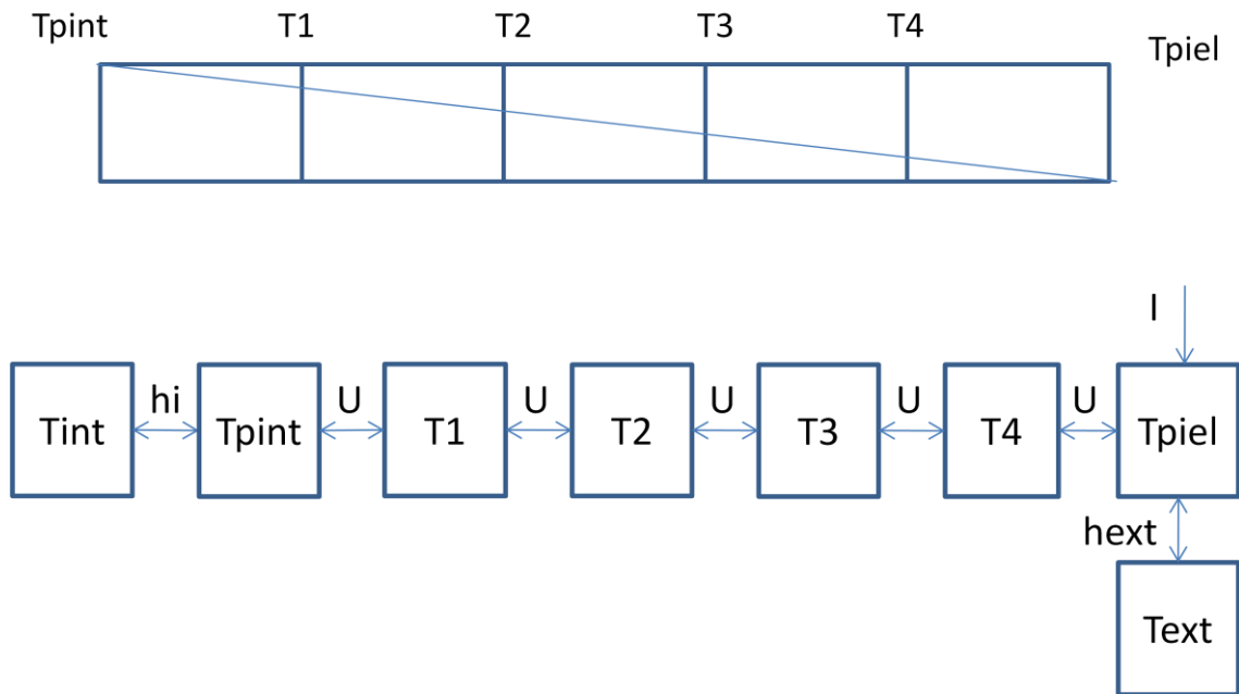
Figura 20. Analogía termoeléctrica.
