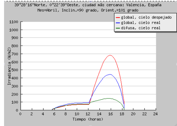
Figura 19. Radiación solar incidente sobre paramento vertical para distintas orientaciones en el mes de Abril en W/m^2 . [5]
