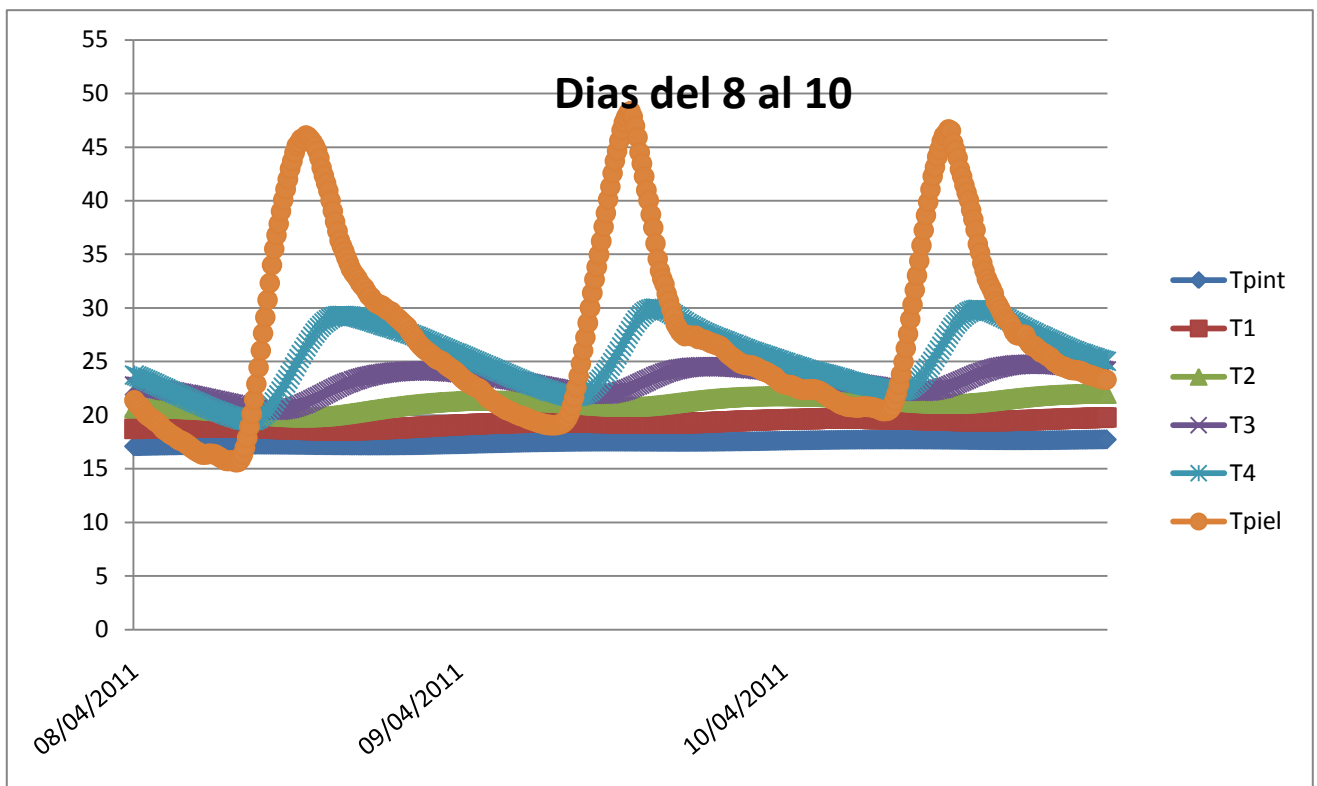
Figura 29. Gráfica de las temperaturas de todas las capas del cerramiento conjuntas del día 8 al 10.
