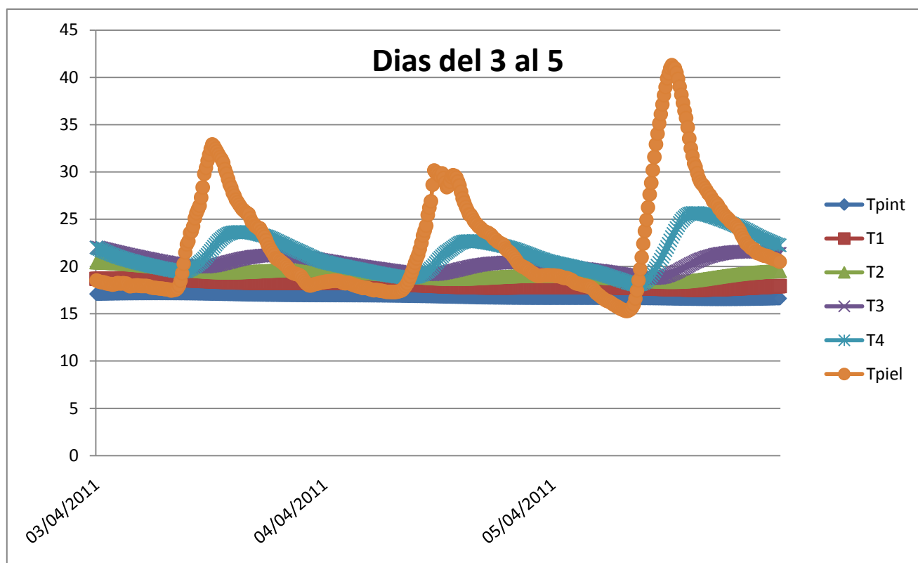
Figura 28. Gráfica de las temperaturas de todas las capas del cerramiento conjuntas del día 3 al 5.
