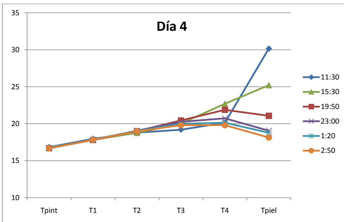
Figura 30. Gráfica del perfil térmico del cerramiento del día 4.
