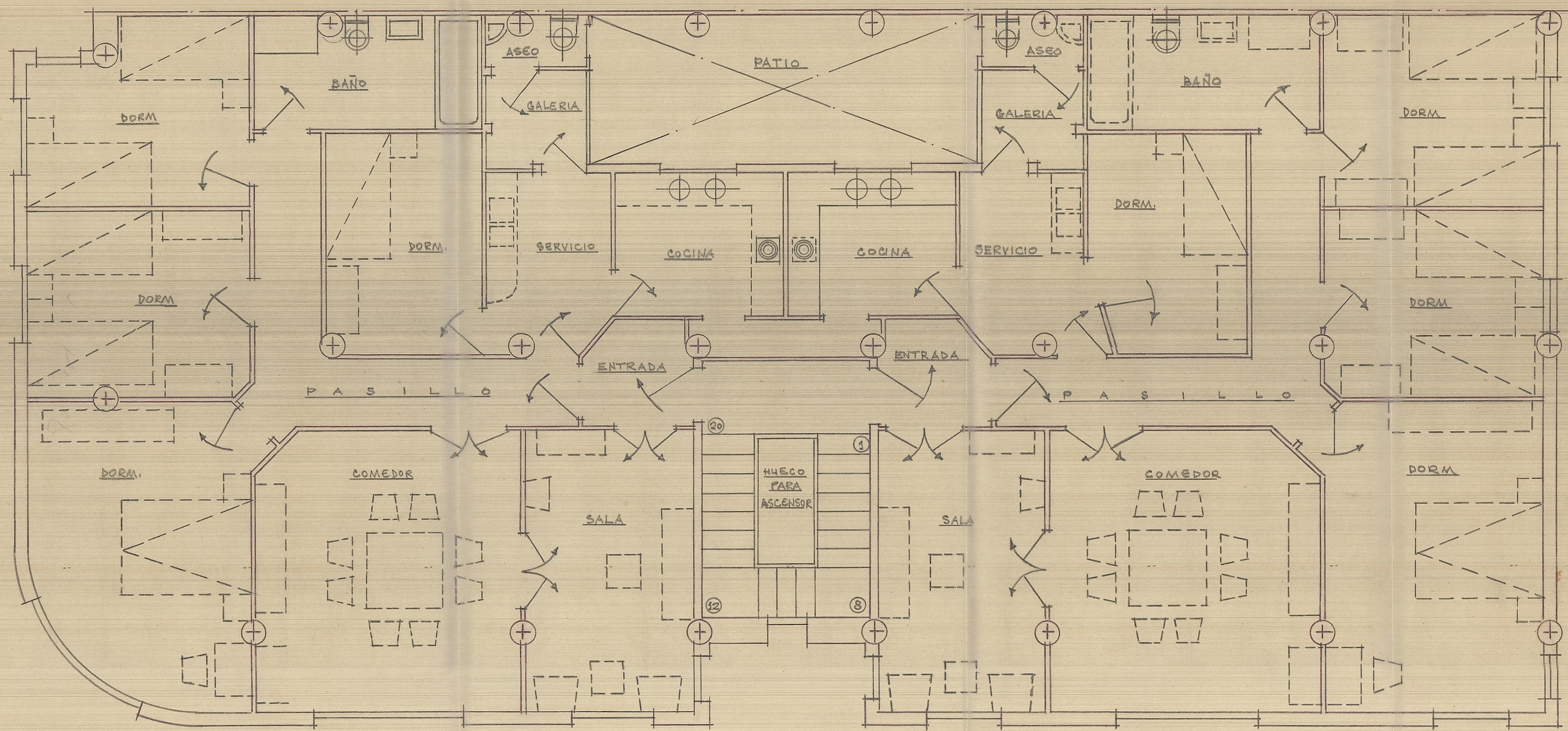
Disposición de las plantas de viviendas
