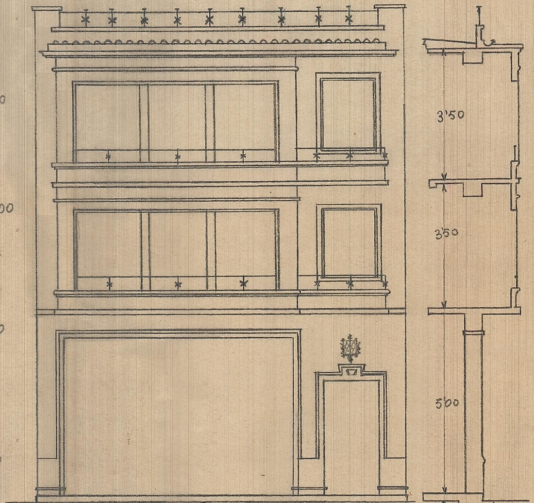
Frente
