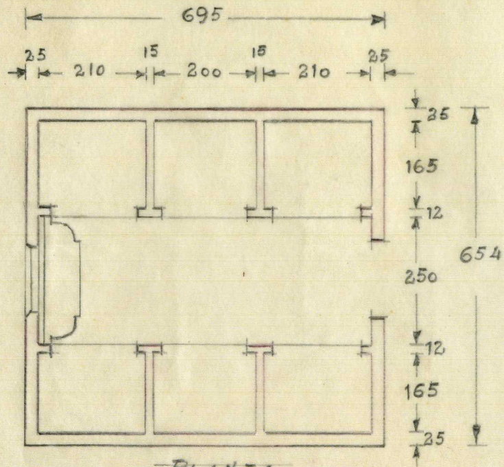
PLANTA
