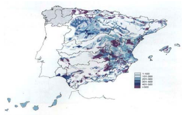
Figura 18. Mapa de capacidad de infiltración máxima (mm)
