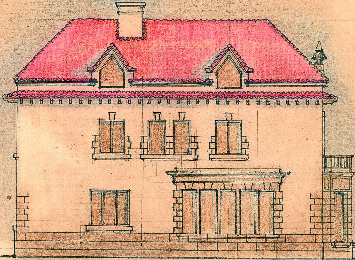
FACHADA OESTE
