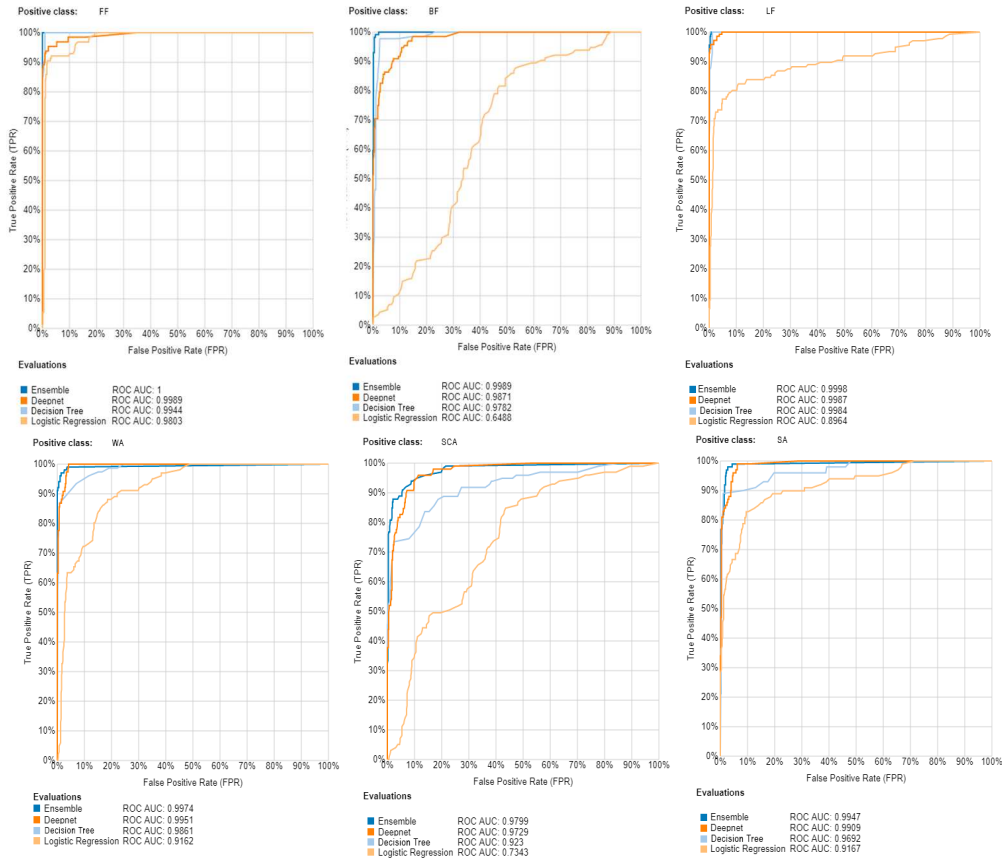
Figura 6.3: Curvas ROC y valores de AUC alcanzados para cada tipo de caída con un promedio de 0.96 (panel superior) y para cada tipo de ADL con un promedio de 0.95 (panel inferior).
