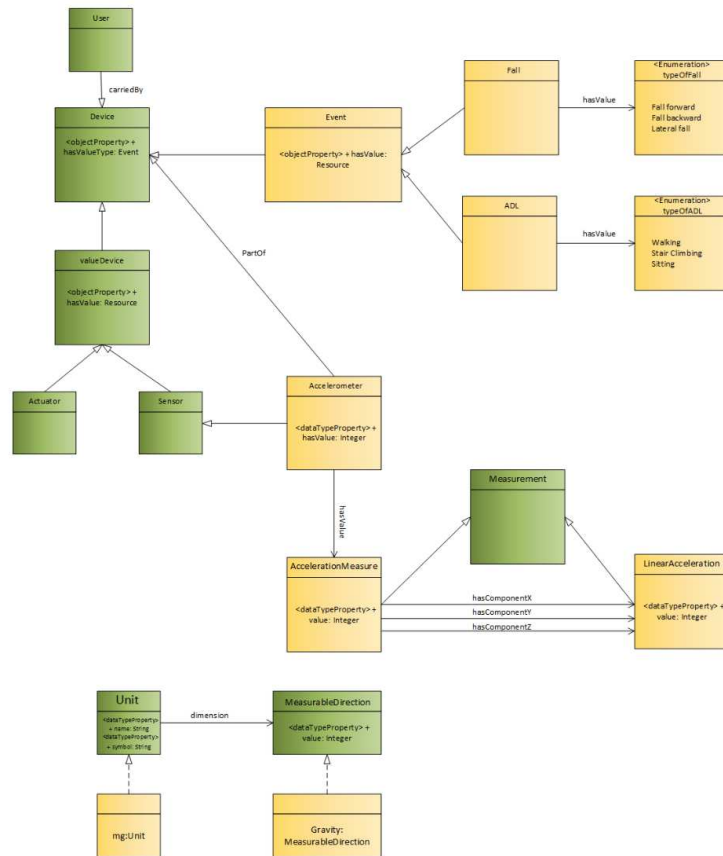
Figura 6.8: Ontología extendida (Device) de UniverSAAL para la representación semántica de los eventos de caídas y actividades
