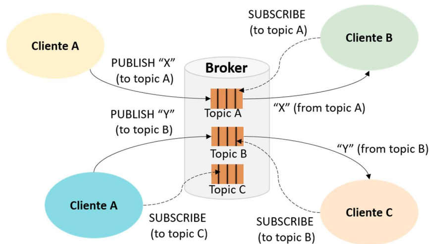
Figura 2.19: Funcionamiento del Protocolo MQTT.
