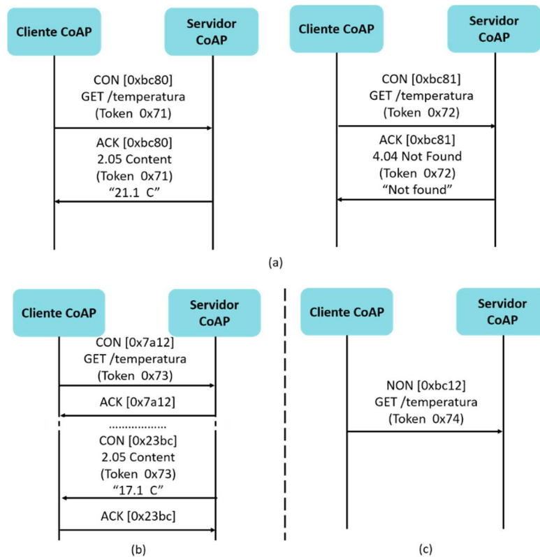
Figura 2.18: Tipos de Mensajes (a) Confirmable con respuesta piggybacked ; (b) Confirmable con respuesta separate (c) No-confirmable.
