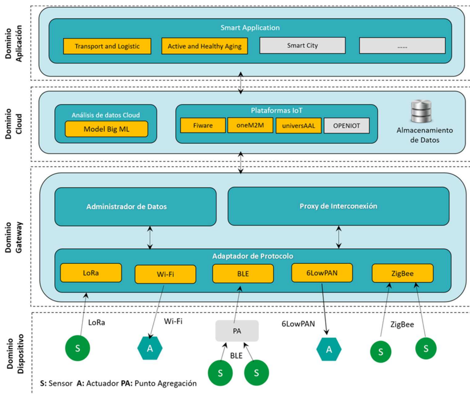
Figura 3.2: Arquitectura de interoperabilidad
