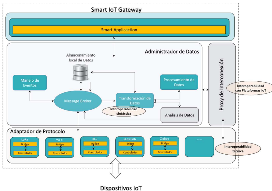
Figura 4.1: Versión embrionaria “ Smart IoT gateway ” de la arquitectura
