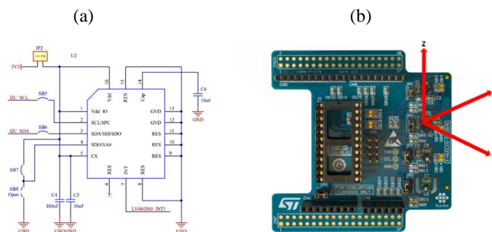
Figura 6.5: Dispositivo portátil (a) Diagrama esquemático; (b) Estructura de hardware
