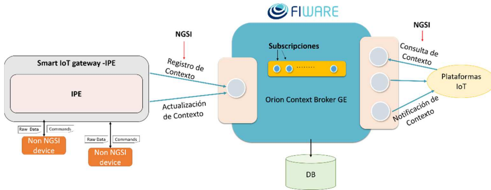
Figura 5.11: Esquema de interconexión con la plataforma FIWARE
