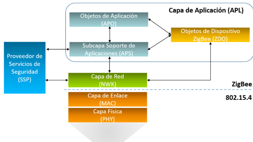
Figura 2.13: Arquitectura ZigBee (Capa de Red y Aplicación)
