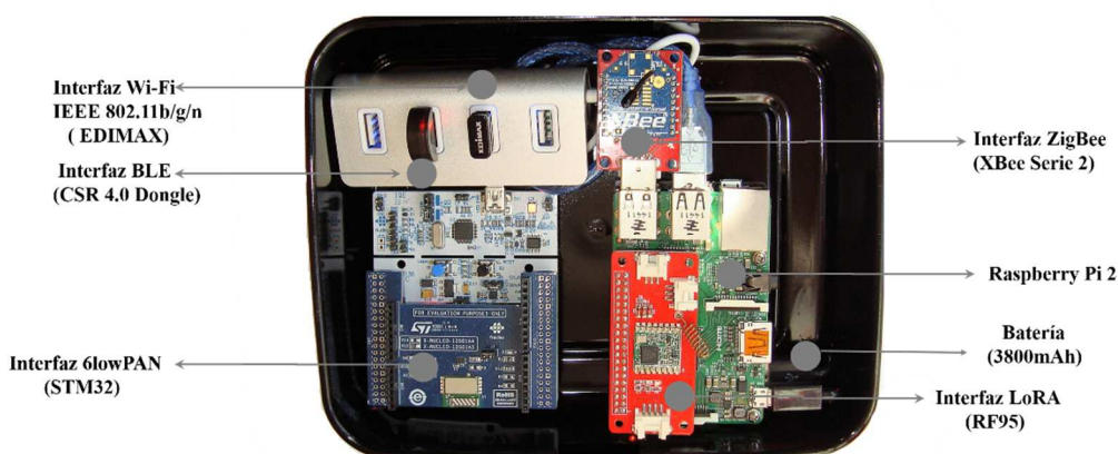
Figura 4.4: Plataforma de desarrollo del smart IoT gateway e interfaces integradas
