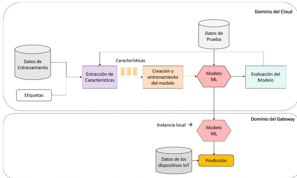
Figura 3.13: Proceso del aprendizaje supervisado ejecutado en el dominio Cloud para crear el modelo ML (parte superior) e instancia local del modelo ML en el dominio del gateway (parte inferior).
