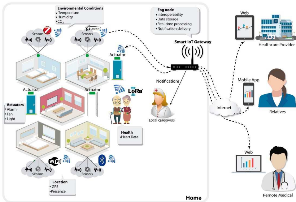
Figura 4.2: Arquitectura del caso de estudio (AAL-IoTSys)
