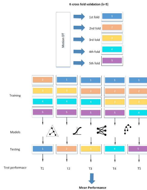
Figura 6.2: Validación cruzada (5-fold) aplicada a Motion-DT para crear y entrenar cada modelo
