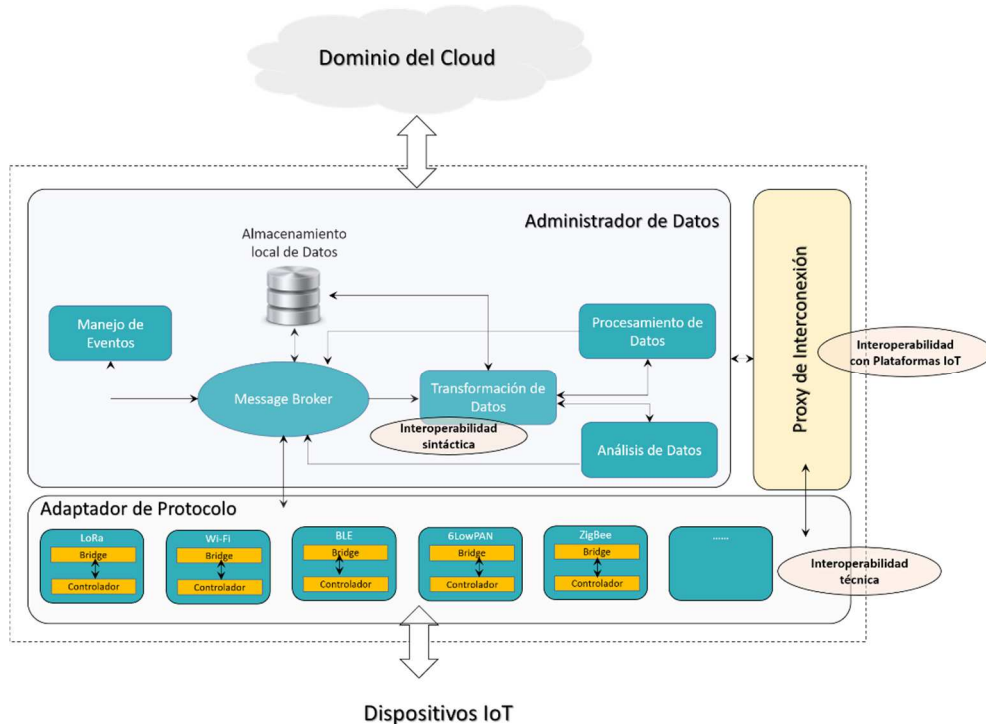
Figura 3.4: Componente Funcional Dominio de Gateway
