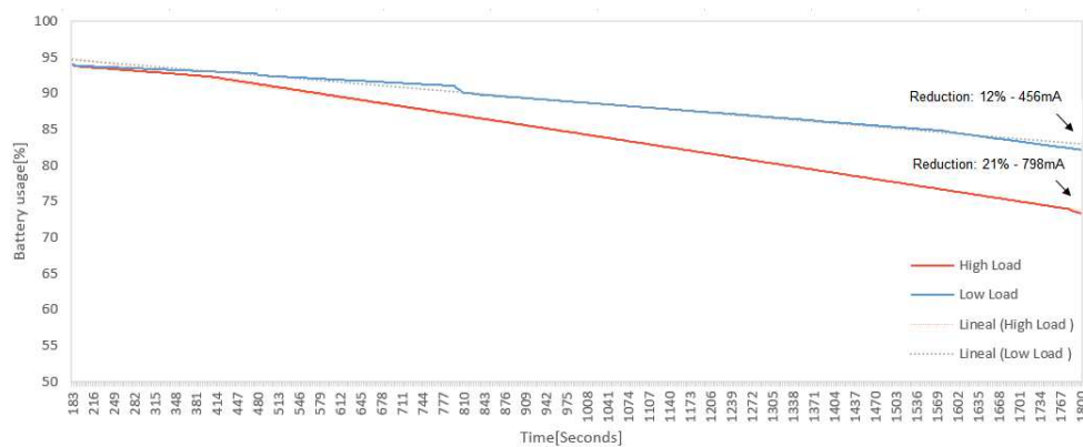
Figura 4.17: Consumo de la batería en los escenarios de carga baja y alta evaluados
