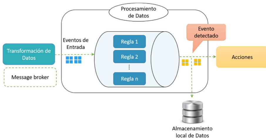
Figura 3.10: Módulo funcional procesamiento de datos
