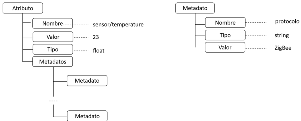
Figura 3.8: Estructura de los atributos y metadatos
