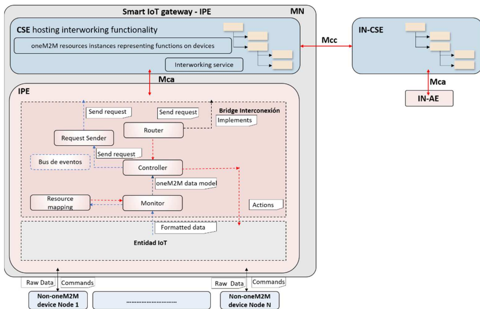
Figura 5.2: Arquitectura de internetworking de dispositivos NoDN con oneM2M basada en IPE
