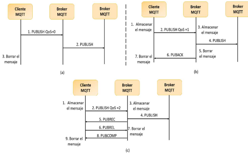
Figura 2.20: Ejemplos de mensajes MQTT utilizando diferentes tipos de QoS
