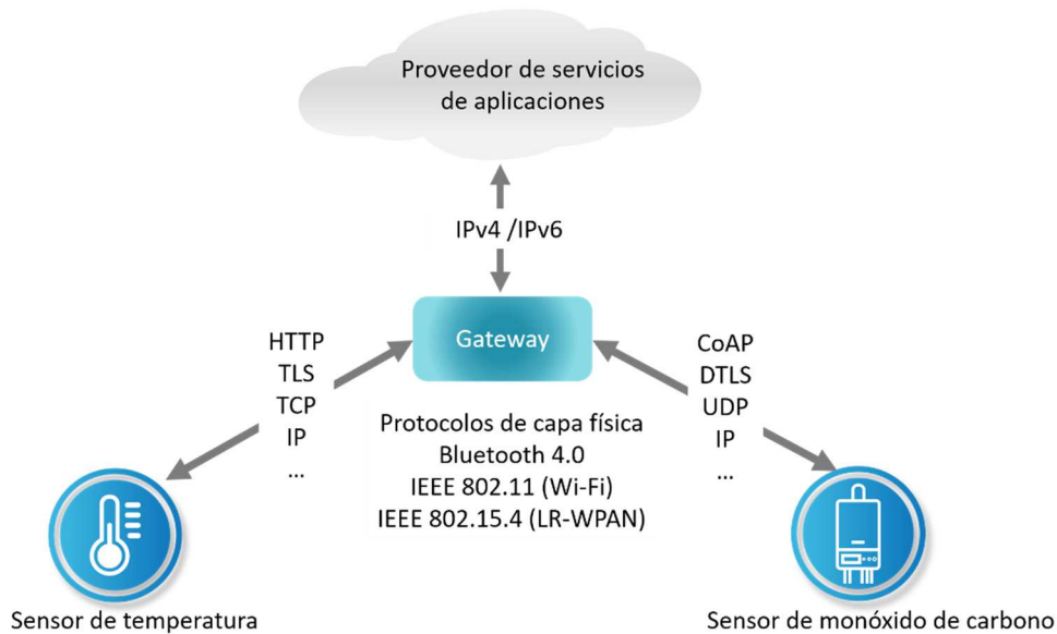
Figura 2.10: Ejemplo del patrón de comunicación D2G.
