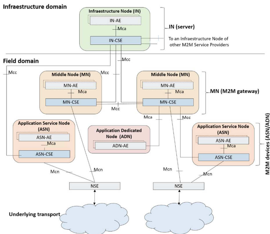
Figura 5.1: Arquitectura funcional oneM2M
