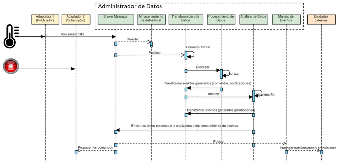
Figura 3.12: Flujo de datos de la arquitectura utilizando el mecanismo publish/subscribe
