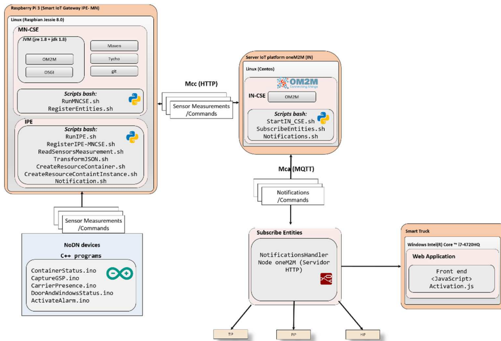
Figura 5.6: Diagrama funcional del testbed implementado
