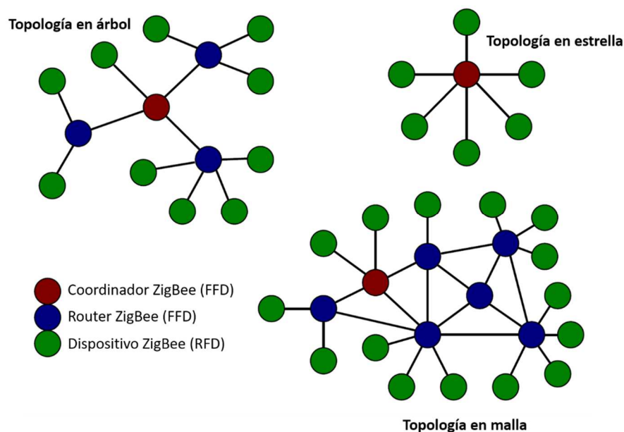
Figura 2.14: Topologías, nodos lógicos y dispositivos soportadas por la tecnología ZigBee
