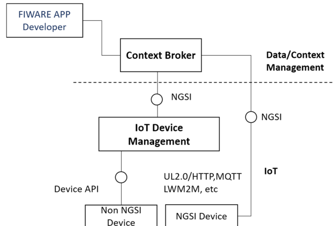
Figura 5.9: Arquitectura IoT de FIWARE
