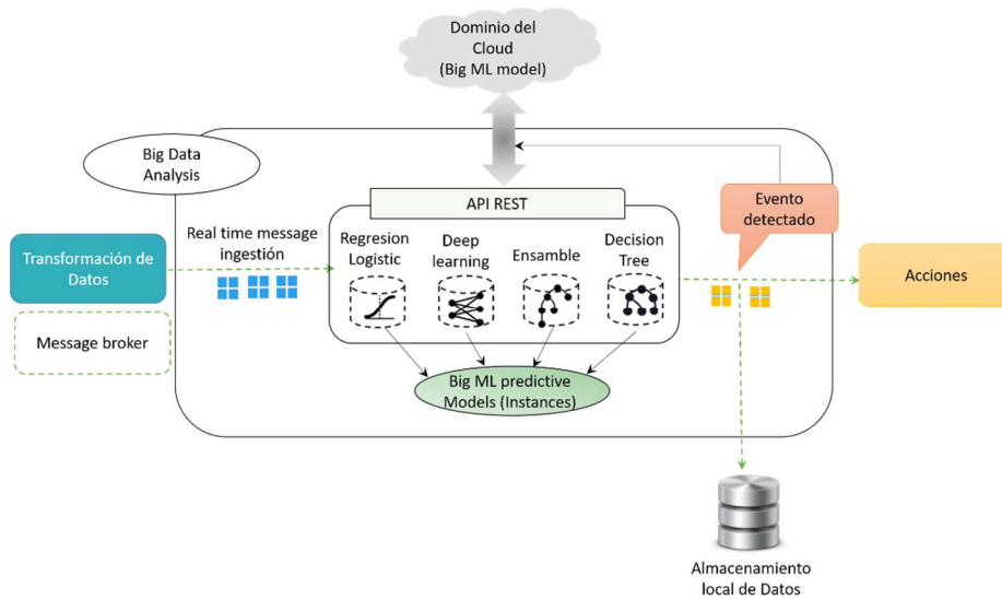
Figura 3.11: Módulo funcional análisis de datos
