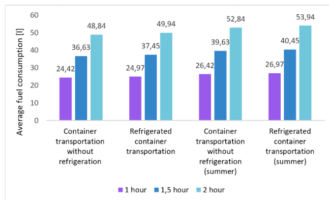
Figura 5.8: Consumo medio adicional de combustible de un camión por viaje
