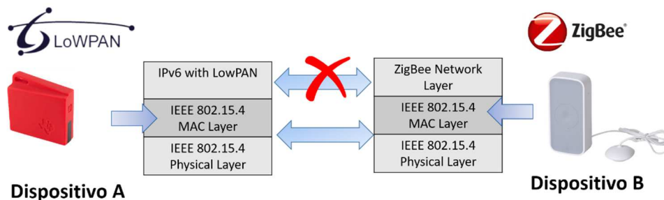
Figura 2.12: Ejemplo de dos dispositivos no interoperables que utilizan el mismo estándar.
