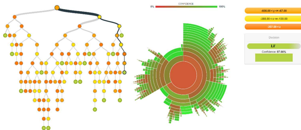
Figura 6.6: Clasificación para uno de los árboles de decisión que forman el ensemble : (izquierda) diagrama del árbol de decisión, (centro) grado de confianza alcanzado por el árbol de decisión al predecir la clase LF, (derecha) regla de decisión generada por el árbol de decisión para predecir la clase LF.
