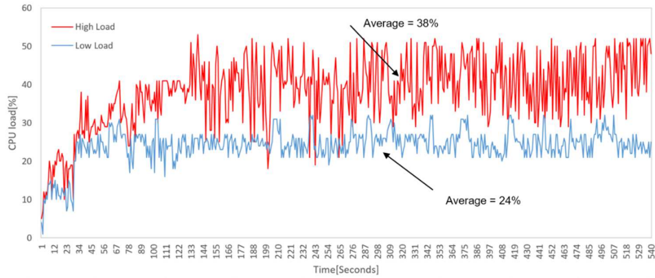
Figura 4.15: CPU promedio del Smart IoT Gateway en los escenarios de carga baja y alta evaluados
