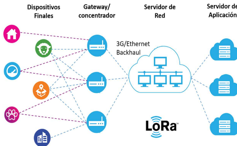
Figura 2.15: Componentes de una red LoRaWAN
