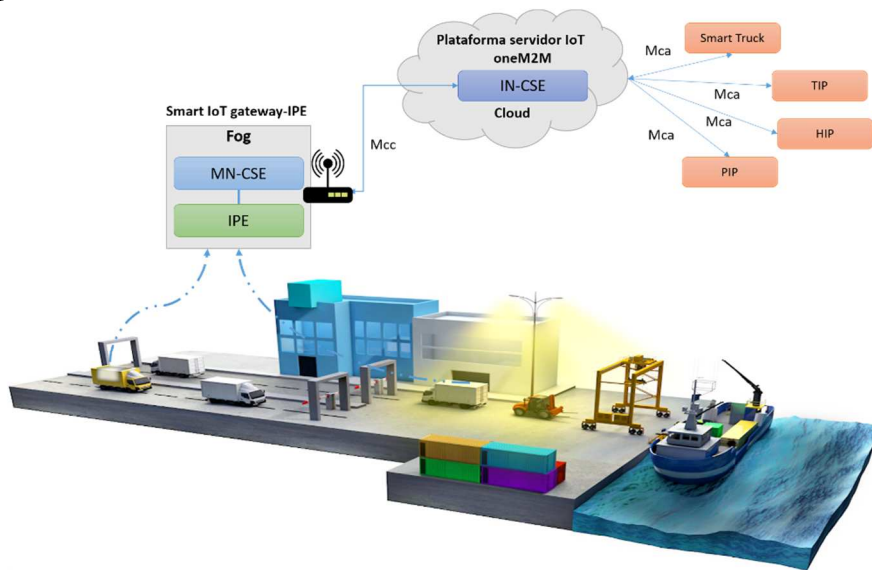
Figura 5.3: Testbed de interconexión
