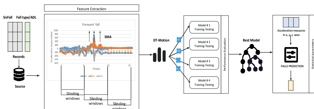
Figura 6.1: Etapas del sistema IoT-E-Fall
