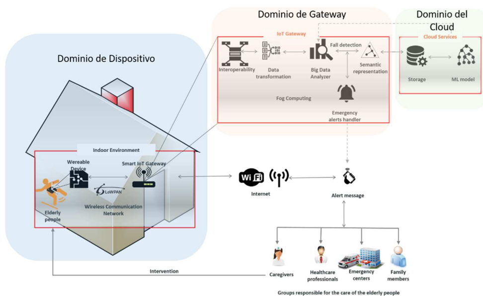
Figura 6.4: Visión general del sistema IoTE-Fall
