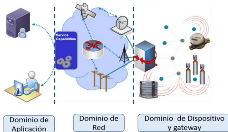
Figura 2.6: Arquitectura M2M ETSI.
