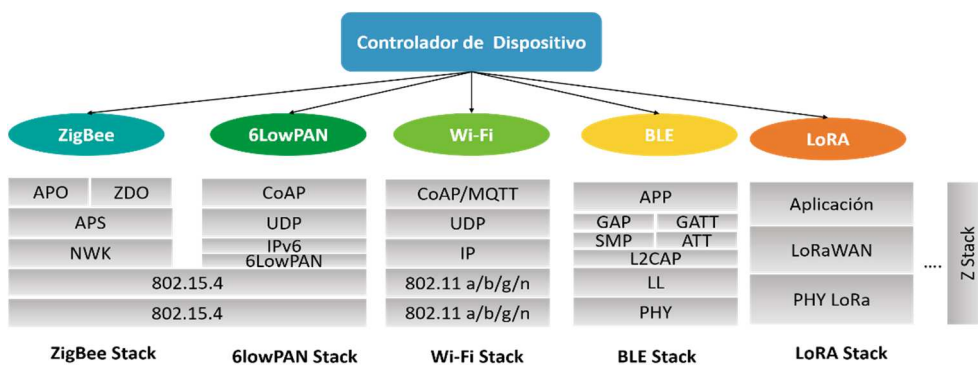
Figura 3.5: Ejemplos de pilas de protocolos de comunicación admitidas por el controlador de dispositivo
