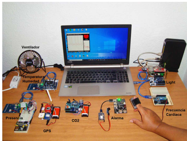
Figura 4.3: Dispositivos IoT utilizados en el prototipo AAL
