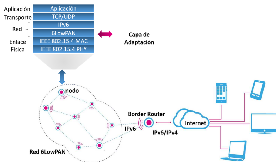
Figura 2.16: Red y pila de protocolos 6lowPAN
