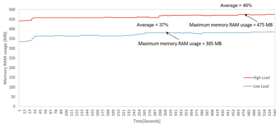
Figura 4.16: Uso de la memoria RAM en los escenarios de carga baja y alta evaluados
