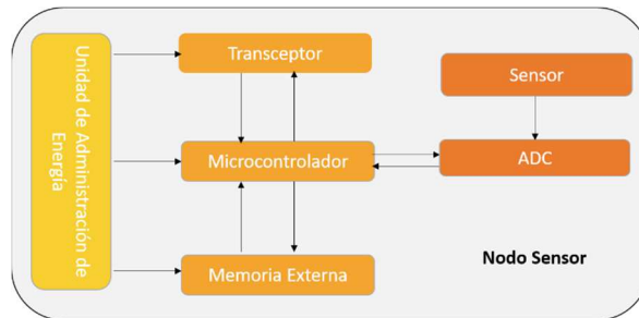
Figura 3.3: Componentes de un dispositivo IoT
