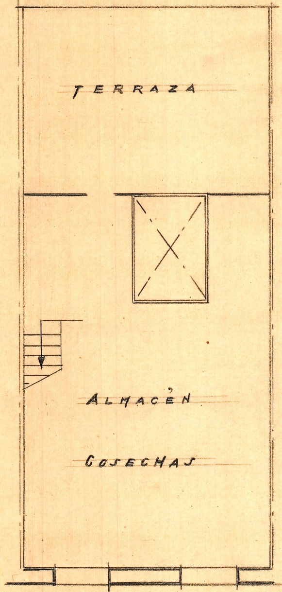
PLANTA ACTUAL
