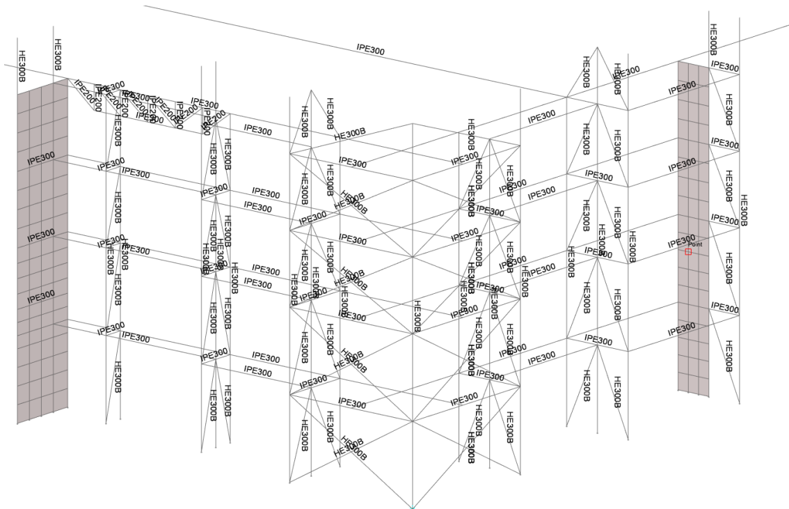
Anexo 1.5 Perfiles de la estructura portante del hall principal
