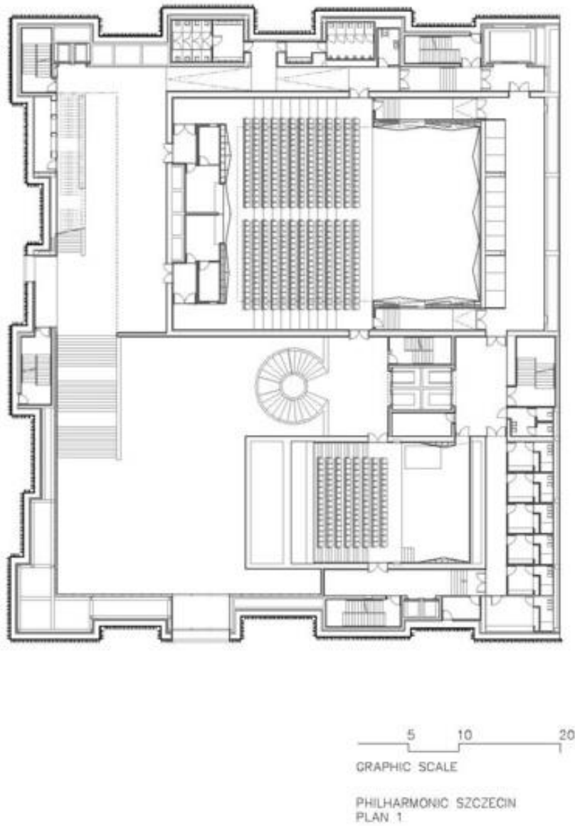
Anexo 2.2 Primera Planta
