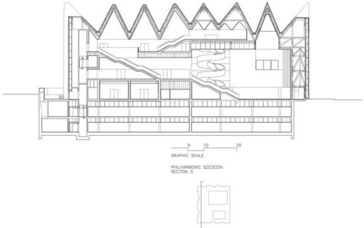
Anexo 2.4 Sección longitudinal
