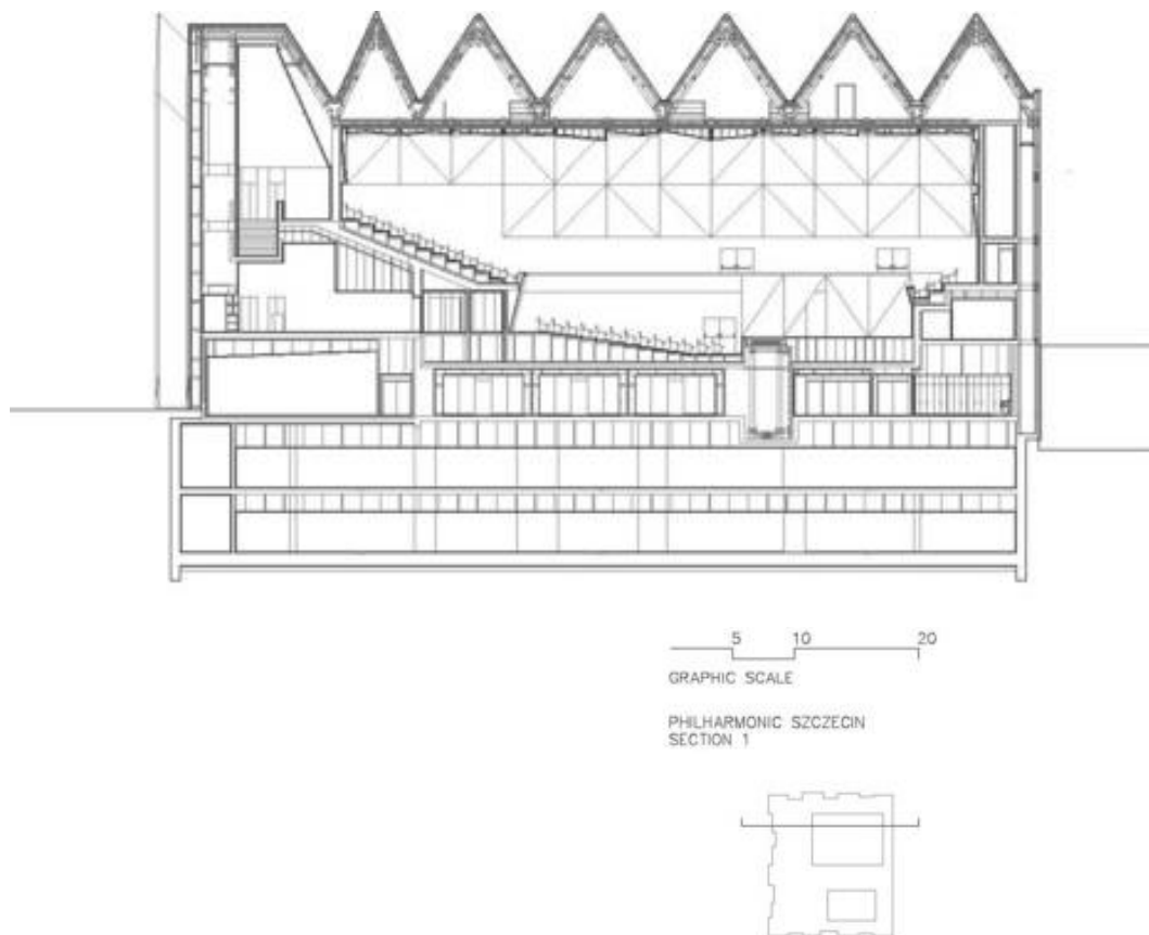
Anexo 2.5 Sección transversal
