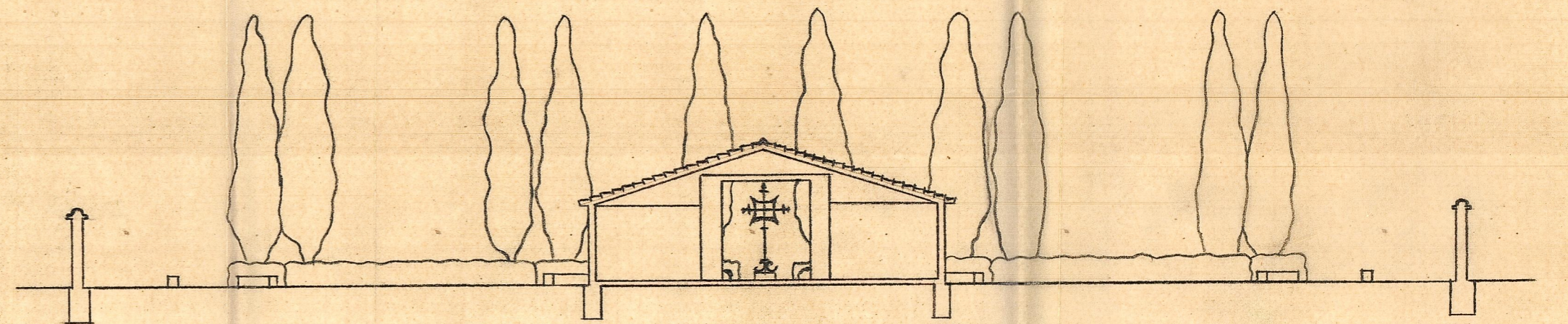
SECCION TRANSVERSAL
