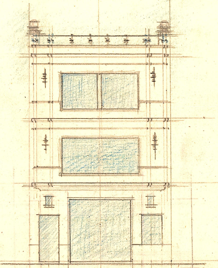
FACHADA A LA CALLE DE SAN FERNANDO
