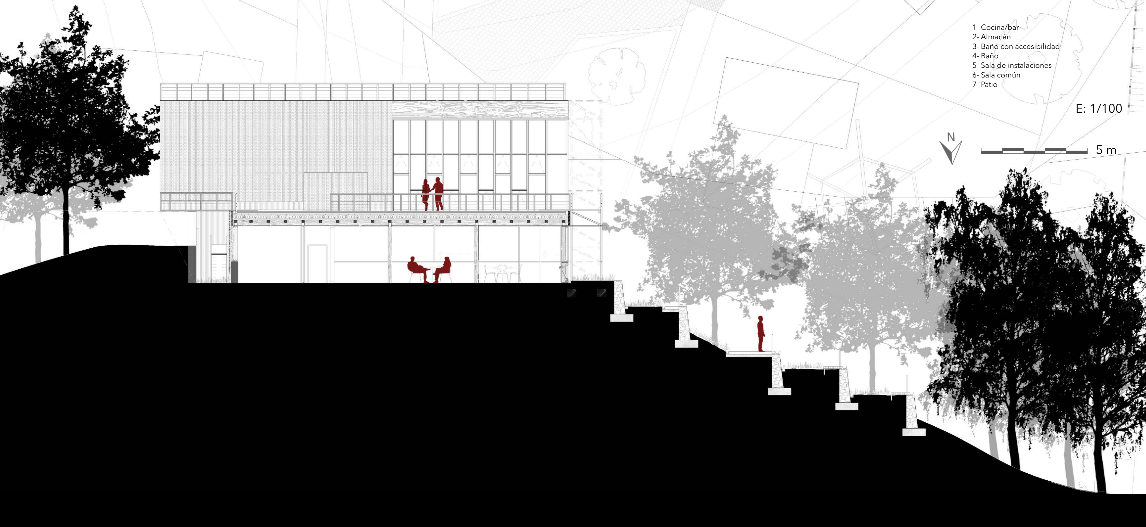
SECCIÓN A-A' E:100
