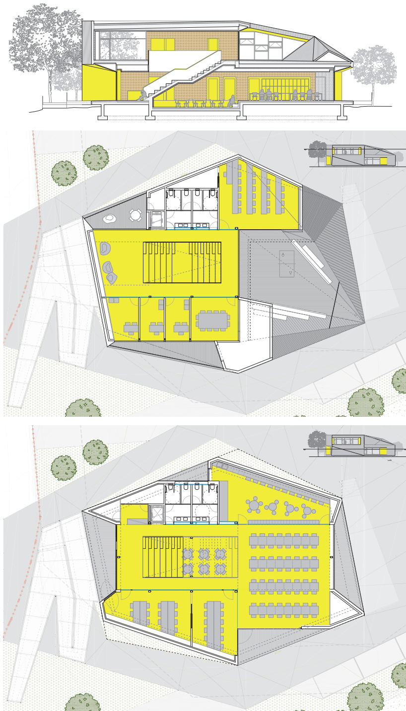
Figure 6. Plants and longitudinal section. Crystalzoo Archive © (2019) / Figura 6. Plantas y seccion longitudinal. Archivo Crystalzoo© (2019).
