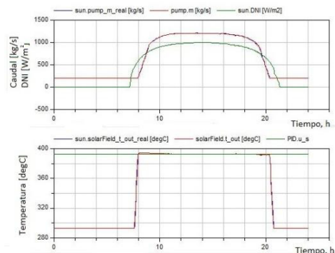
Figura 19: Control de temperatura del campo solar en un día soleado
