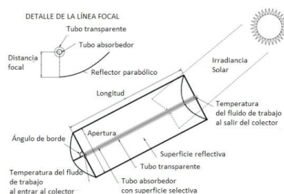
Figura 6: Esquema de un colector solar cilindro-parabólico
