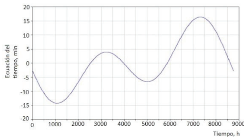
Figura 4: Variación anual de la corrección del tiempo
