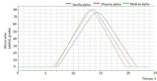
Figura 14: Comparativa de la altura solar entre Sevilla, Phoenix y Madras
