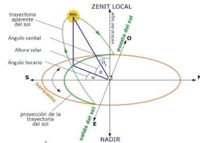
Figura 5: Ángulos que definen la posición del sol
