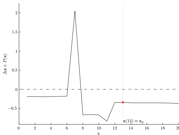
Figura 9: Estudio de estabilidad de la oscilación localizada.
