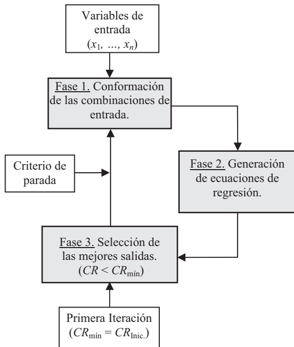
Figura 1: Fases del proceso de diseño del algoritmo GMDH.
