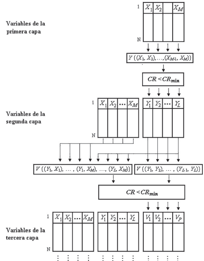
Figura 6: Representación generalizada del diseño de una red neuronal GMDH.
