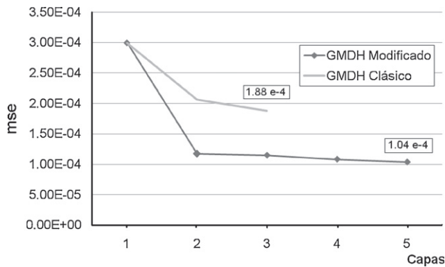
Figura 14: Convergencia del error durante el entrenamiento.
