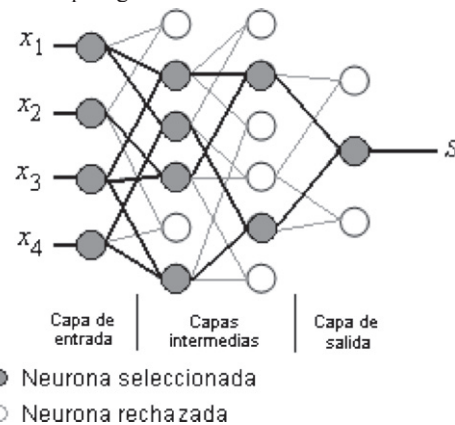
Figura 2: Ejemplo de estructura de red neuronal obtenida mediante algoritmo GMDH.
