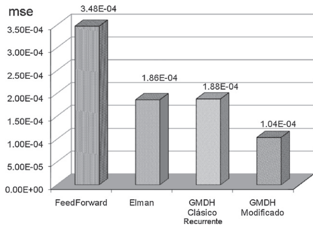
Figura 16: Comparación aplicando diferentes modelos neuronales al caso de estudio.
