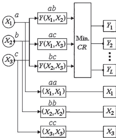
Figura 5: Diagrama de conformación del conjunto de variables que pasan a la siguiente capa.
