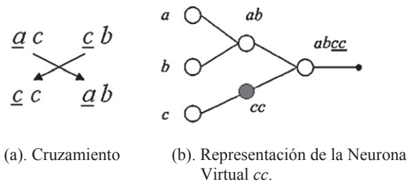
Figura 4: Ejemplo de neurona virtual obtenida por cruzamiento.
