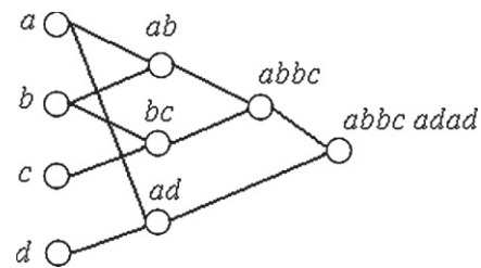
Figura 3: Ejemplo de codificación donde se representa una neurona virtual.
