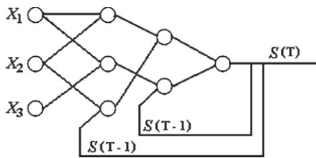
Figura 7: Ejemplo de formación de un lazo recurrente en cada capa intermedia.
