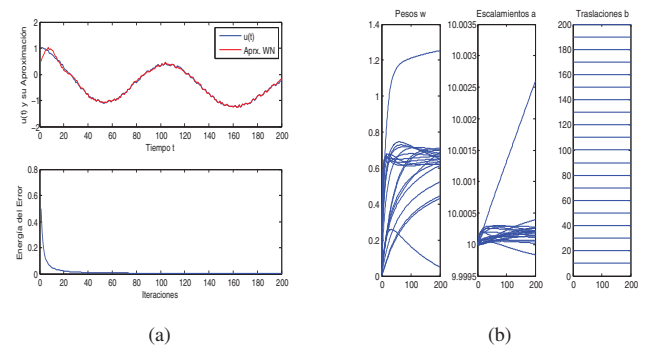
Figura 14: Aproximación Wavenet de la Función u(t) = -\frac{0.35}{100}t + cos(\frac{t}{17})e^{-\frac{t}{400}} + ruido con 20 Neuronas y Wavelet Morlet (a). La Actualización de los Parámetros Durante el proceso de Aprendizaje (b).
