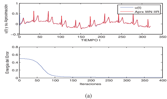
Figura 21: Aproximación Wavenet de un ECG y la Energía del Error (a). La Actualización de los Parámetros de la Red Durante el Proceso de Aprendizaje (b).
