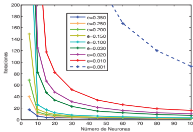
Figura 12: Iteraciones Requeridas por las Wavenets para Diferentes Valores de K con Respecto a Diferentes Umbrales de Error, para una señal de entrada u(t) = exp(-t/50) * sin(t/5) + ruido
