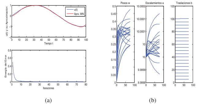
Figura 10: Aproximación Wavenet con K = 20 y su Función de Energía (a). La Actualización de los Parámetros Durante el proceso de Aprendizaje (b).
