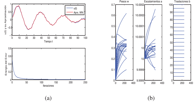
Figura 13: Aproximación Wavenet de la Función u(t) = e^{-t/50} sin(\frac{t}{5}) + ruido con 20 Neuronas y Wavelet Morlet (a). La Actualización de los Parámetros Durante el proceso de Aprendizaje (b).
