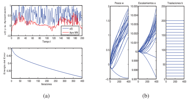
Figura 6: Aproximación Wavenet con 20 Neuronas y Wavelet SLOG2, y su Función de Energía (a). La Actualización de los Parámetros Durante el Proceso de Aprendizaje (b).
