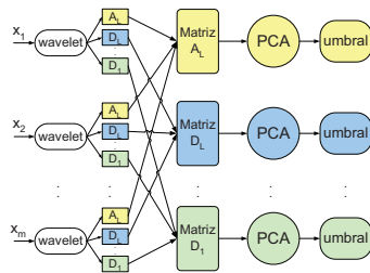
Figura 9: Esquema del cálculo de PCA en el método MSPCA.
