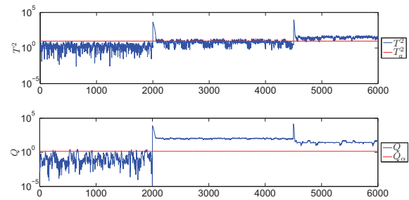
Figura 3: Monitorización de dos fallos con PCA.
