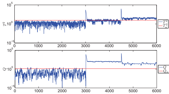
Figura 17: Monitorización de dos fallos con PCAEA.
