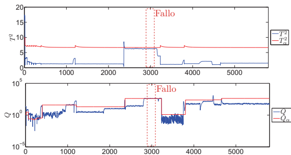
Figura 15: Monitorización de un fallo con EWPCA sobre un protocolo de funcionamiento con varios modos de operación.
