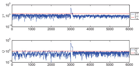
Figura 5: Monitorización de un fallo con APCA.
