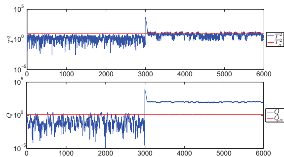
Figura 19: Monitorización de un fallo con PCANLEA.
