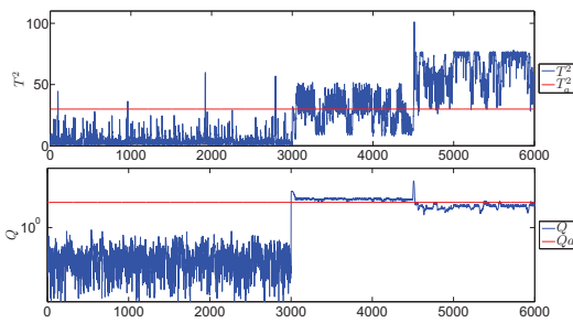
Figura 24: Monitorización de dos fallos con NLPCA
