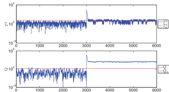
Figura 16: Monitorización de un fallo con PCAEA.
