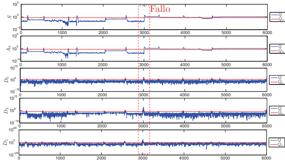
Figura 12: Monitorización de un fallo con MSPCA sobre un protocolo de funcionamiento con varios modos de operación.
