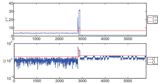
Figura 13: Monitorización de un fallo con EWPCA.
