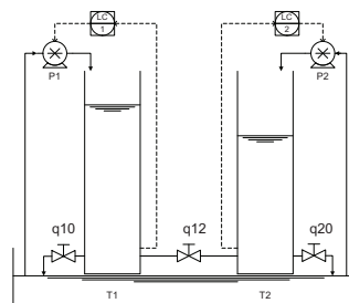
Figura 1: Esquema de la planta piloto.
