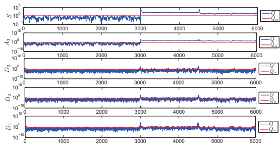
Figura 11: Monitorización de dos fallos con MSPCA.
