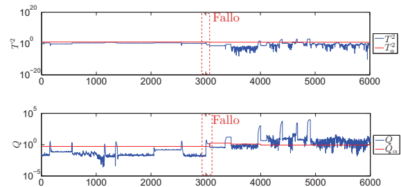
Figura 7: Monitorización de un fallo con APCA sobre un protocolo de funcionamiento con varios modos de operación.
