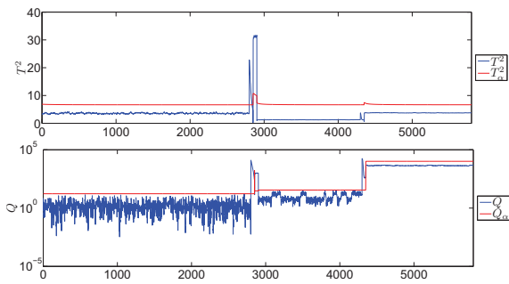
Figura 14: Monitorización de dos fallos con EWPCA.
