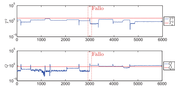
Figura 4: Monitorización de un fallo con PCA sobre un protocolo de funcionamiento con varios modos de operación.
