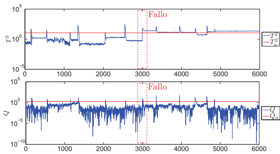
Figura 18: Monitorización de un fallo con PCAEA sobre un protocolo de funcionamiento con varios modos de operación.
