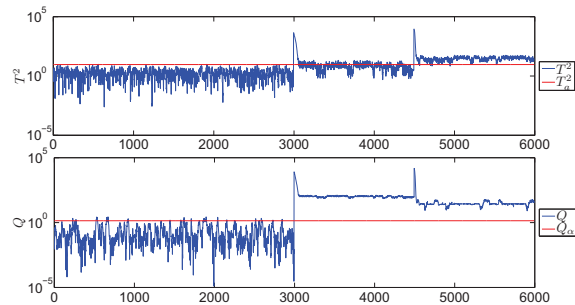
Figura 20: Monitorización de dos fallos con PCANLEA.
