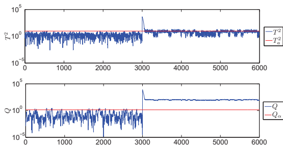
Figura 2: Monitorización de un fallo con PCA.
