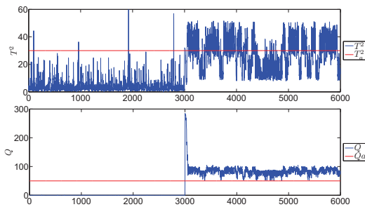
Figura 23: Monitorización de un fallo con NLPCA
