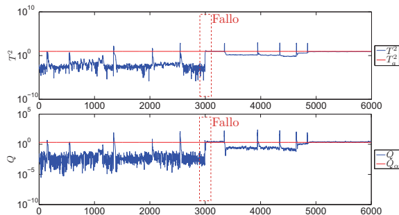
Figura 21: Monitorización de un fallo con PCANLEA sobre un protocolo de funcionamiento con varios modos de operación.
