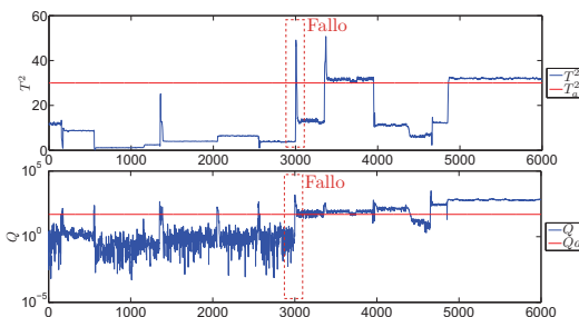
Figura 25: Monitorización de un fallo con NLPCA sobre un protocolo de funcionamiento con varios modos de operación
