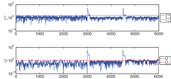
Figura 6: Monitorización de dos fallos con APCA.
