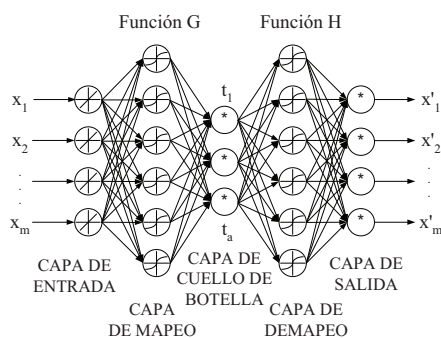
Figura 22: Estructura de red autoasociativa para PCA no lineal
