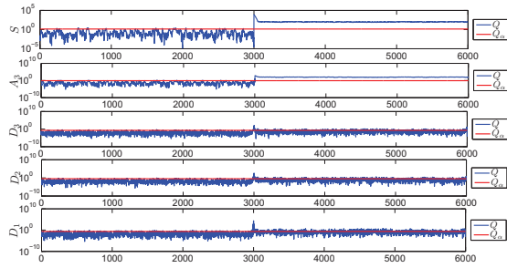
Figura 10: Monitorización de un fallo con MSPCA.
