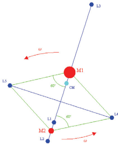
Figura 2. Sistema teórico binario con sus cinco puntos de Lagrange.
