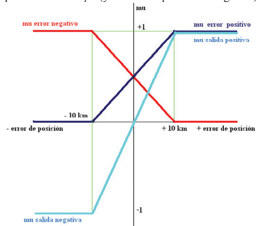
Figura 13: Conjuntos borrosos definidos para las variables de entrada y salida, en las direcciones X e Y del plano.
