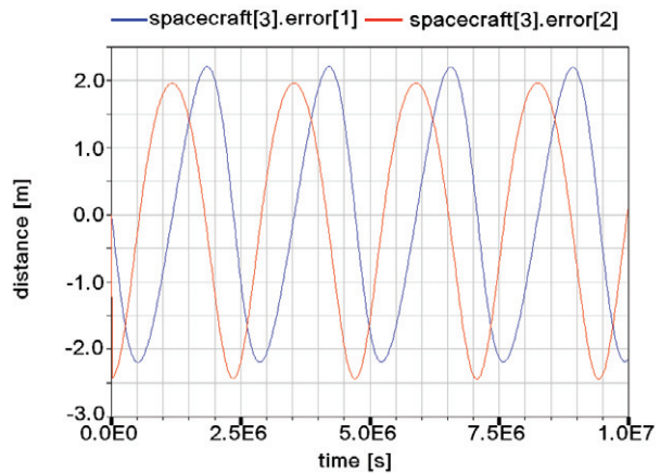
Figura 16: Errores de posición del satélite con control PD borroso en L3.
