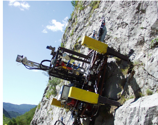
Figura 1. Roboclimber, robot escalador para consolidación de laderas de montañas (CSIC)
