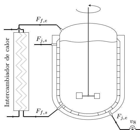
Figura 2. Diagrama de la planta piloto con los cuatro elementos: reactor, intercambiador de calor, camisa de refrigeración y válvula de recirculación.
