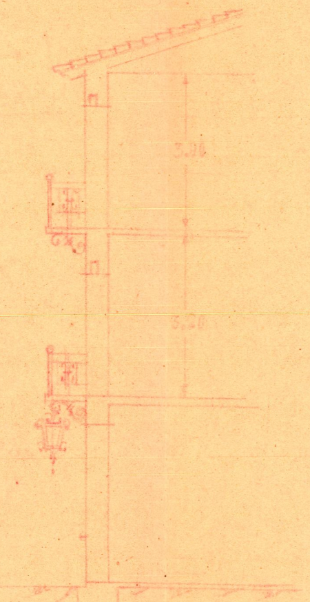
Seccion por A-B
