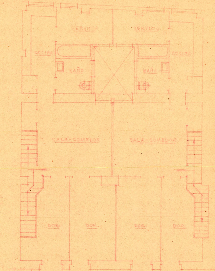
Primer piso Reformado PLANTA
