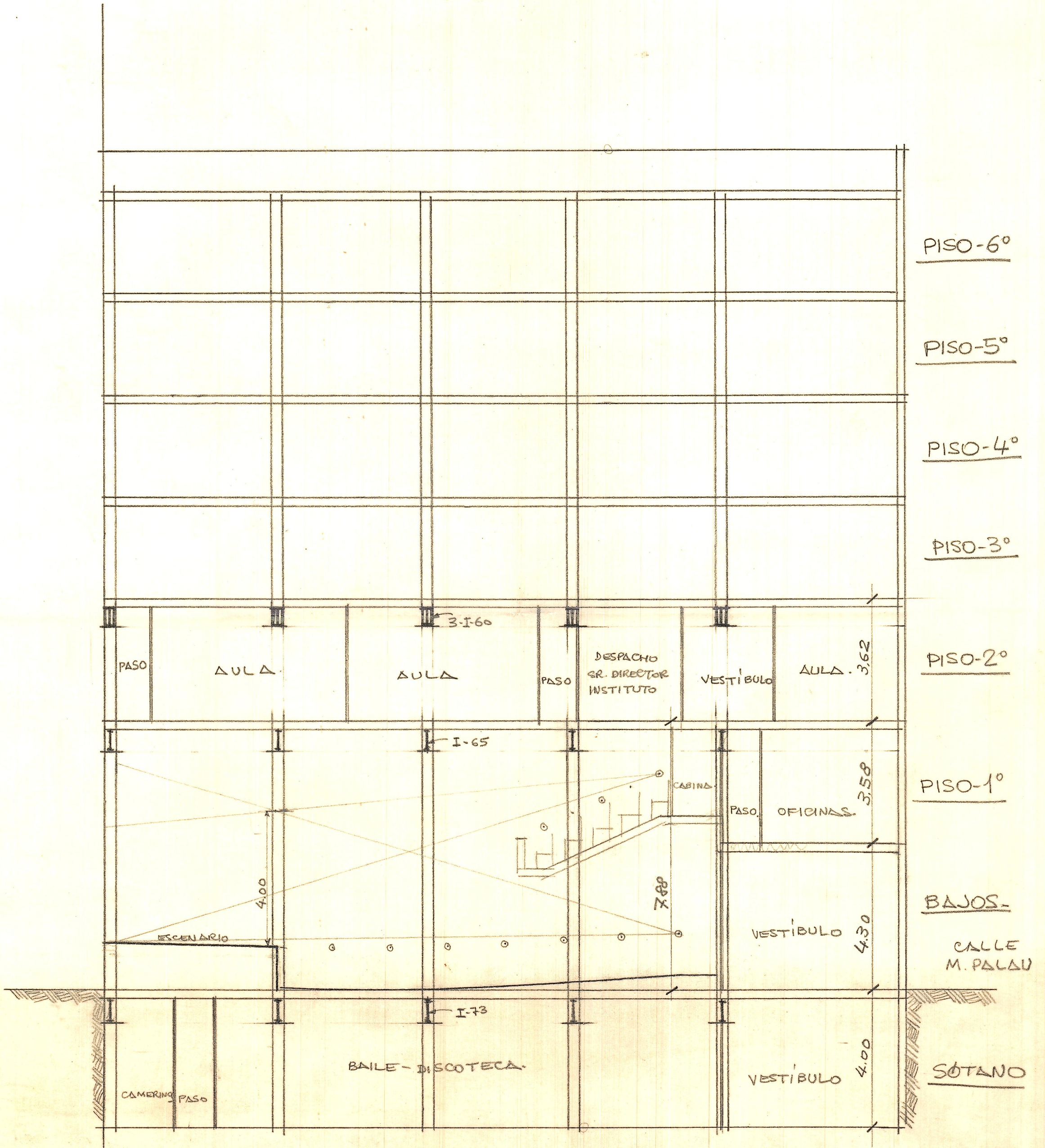
SECCIÓN LONGITUDINAL.
