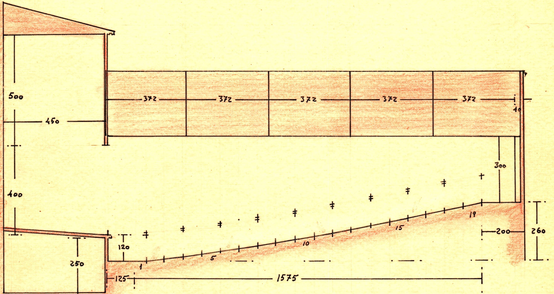
ESCENA INTERIOR - SECCION-E.-1:100
