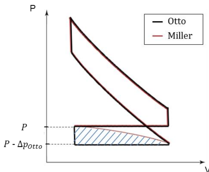
Fig. 4 : « Dethrottling » strategy
